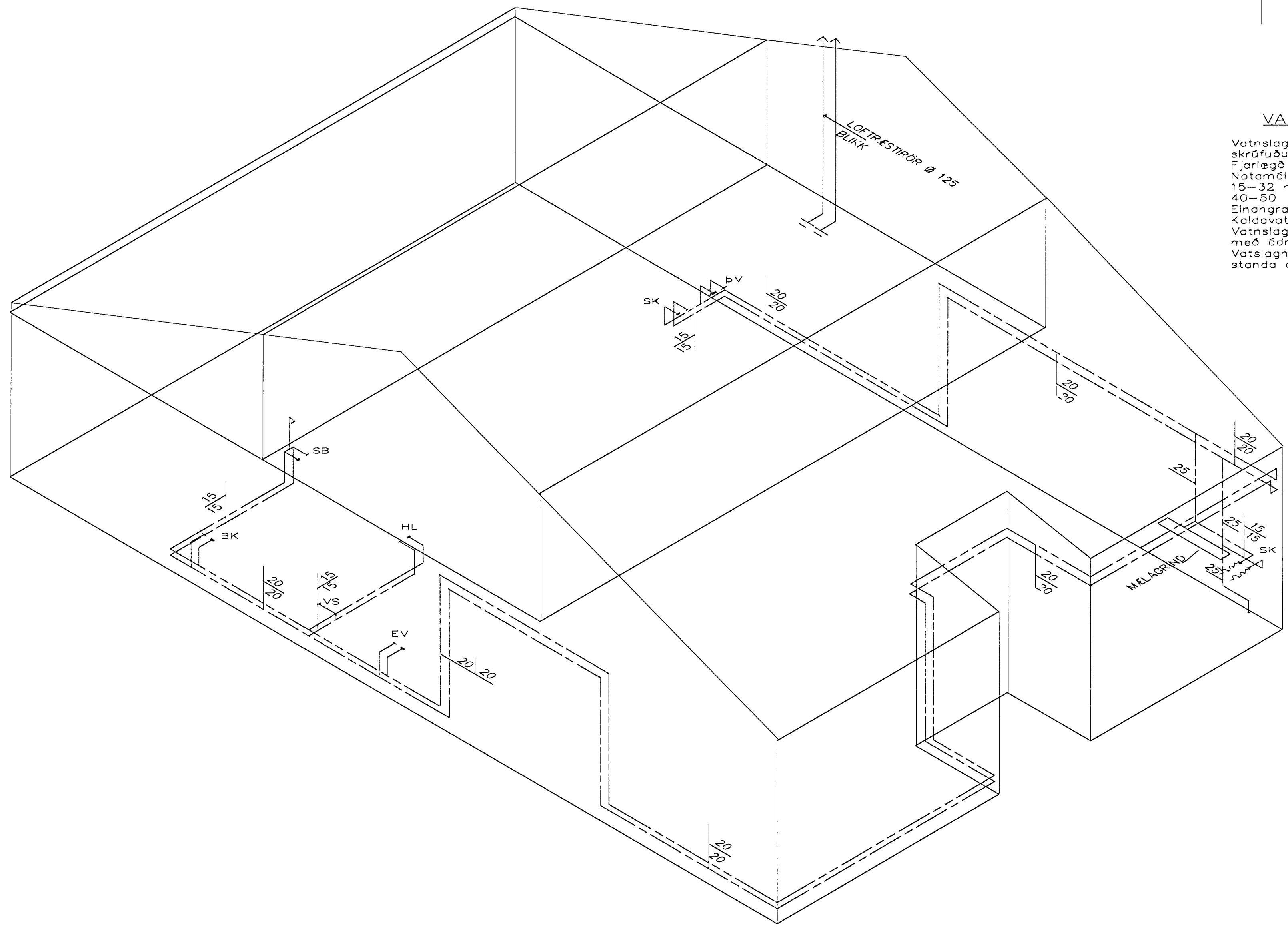
RÜMMYND VATNSLAGNA 1:50
