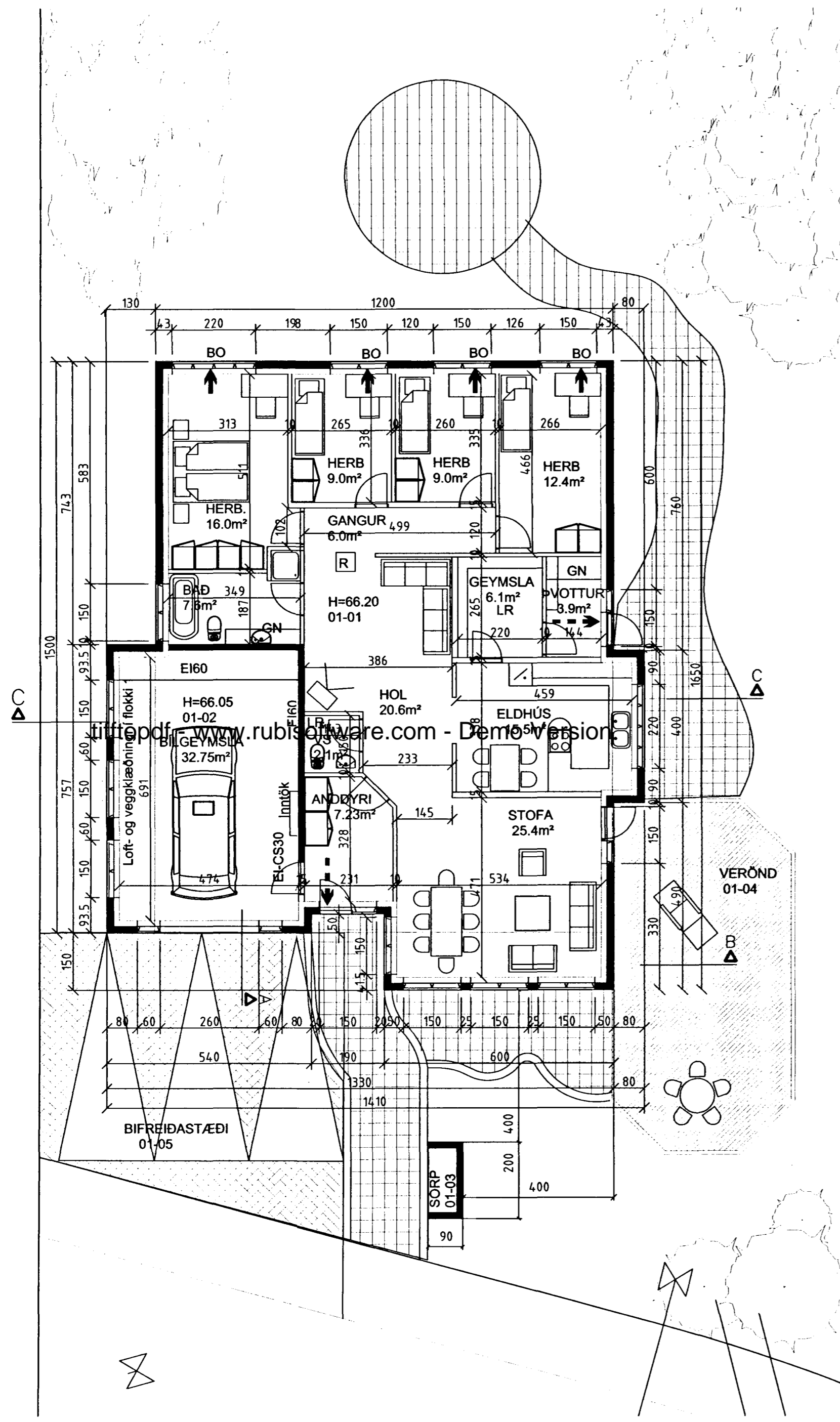
GRUNNMYND MKV. 1:100
