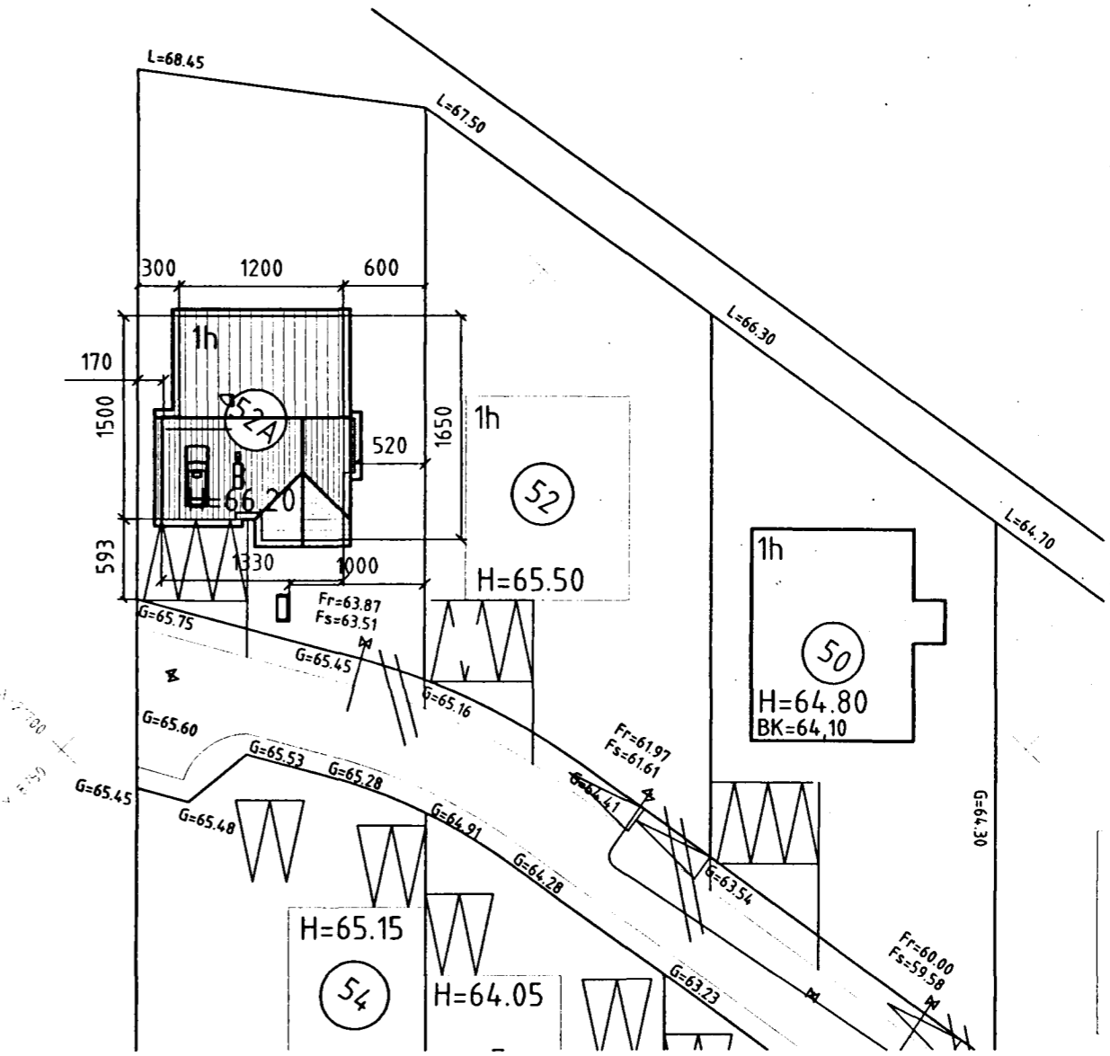
AFSTÖÐUMYND MKV. 1:500
