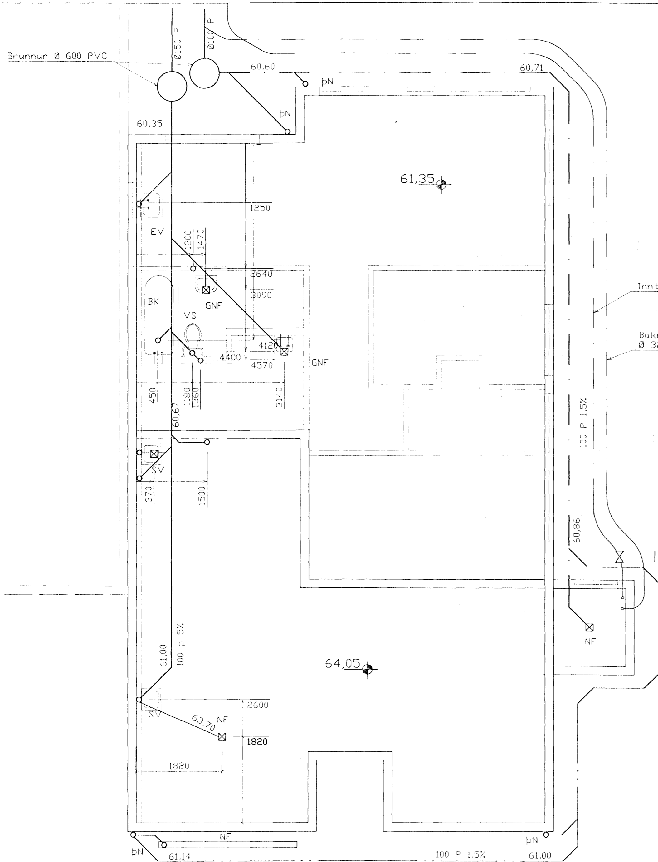
Grunnmynd 1/50
