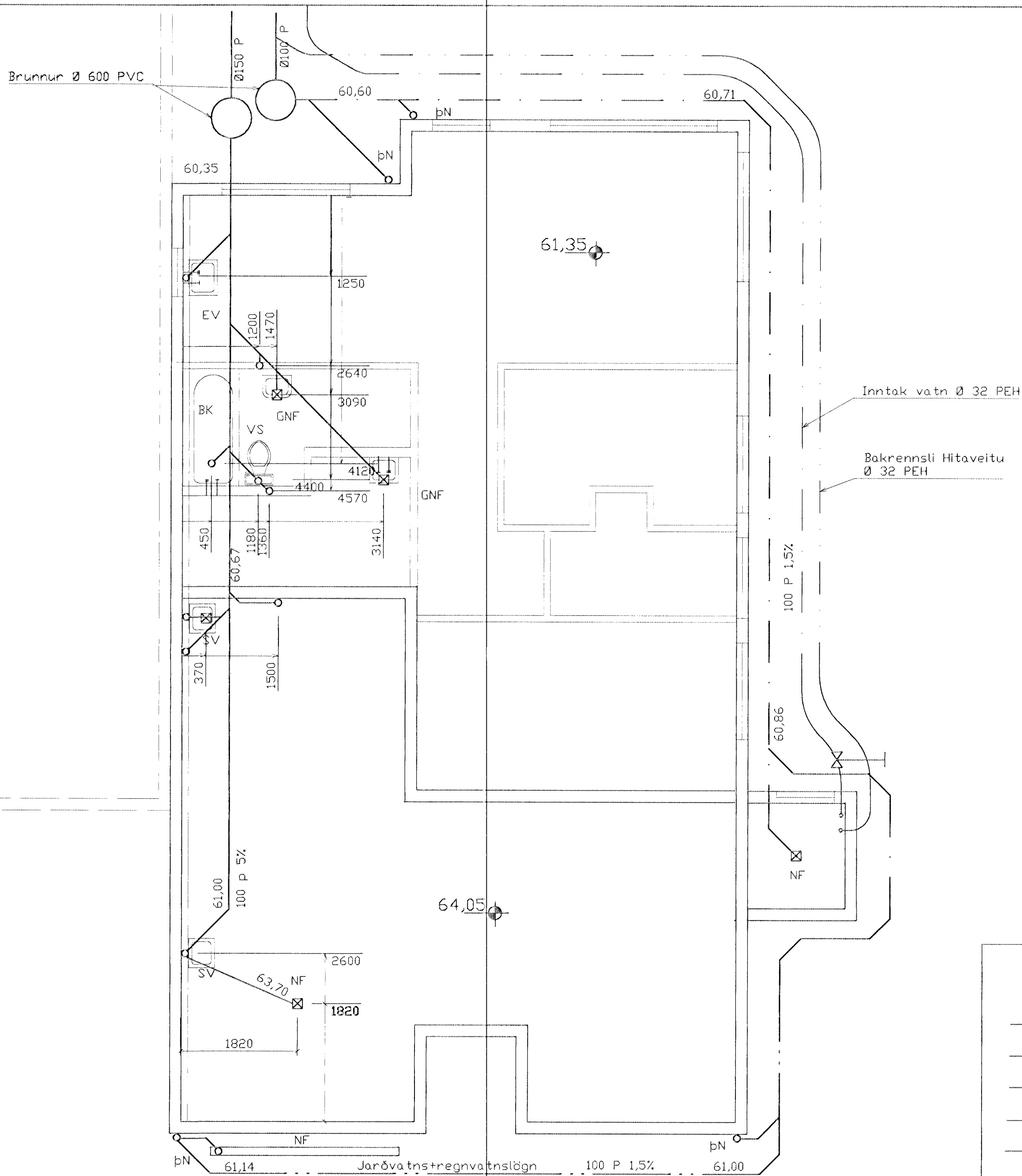
Grunnmynd 1/50
