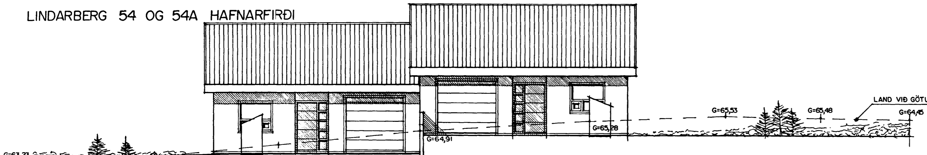
ÚTLIT NORÐAUSTUR MKV. 1:100.
