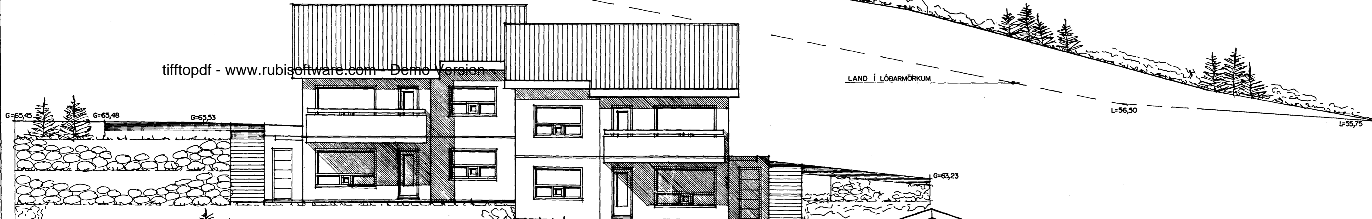
ÚTLIT NORÐVESTUR MKV. 1:100.
