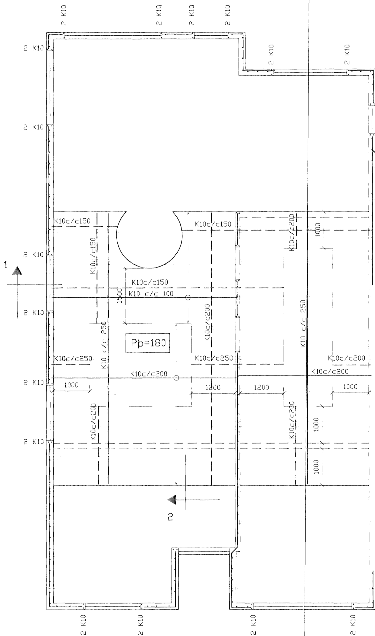
Grunnmynd 1/50
