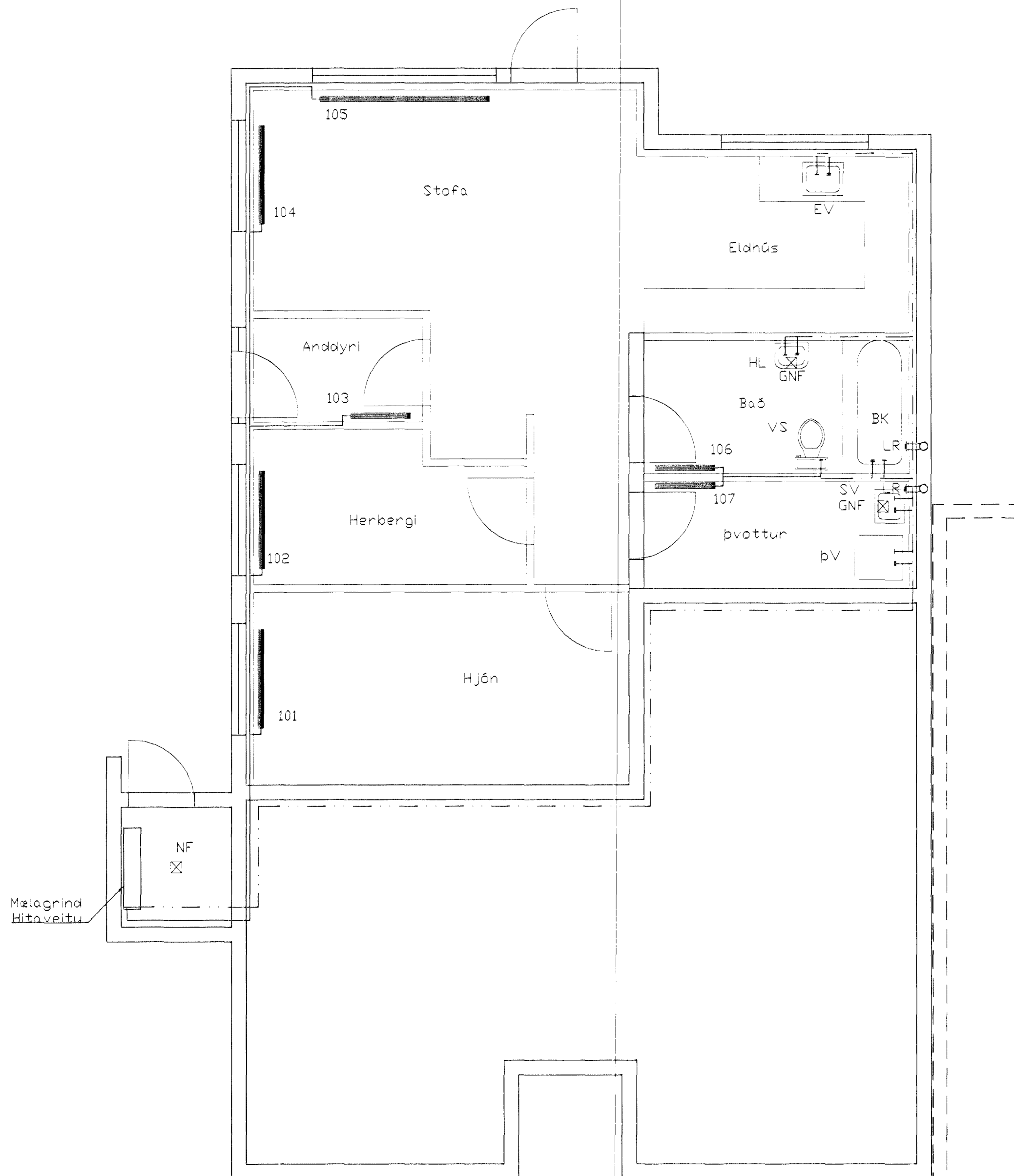
Grunnmynd jarðhæð, 1:50
