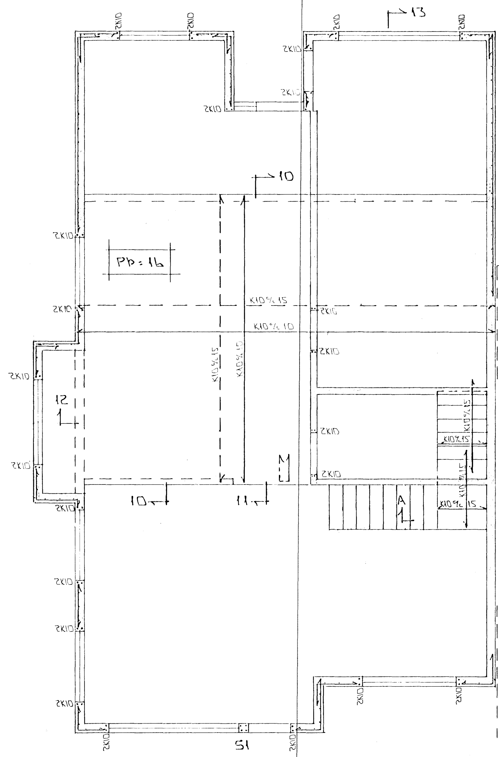
GRUNNMÝND 1:50
