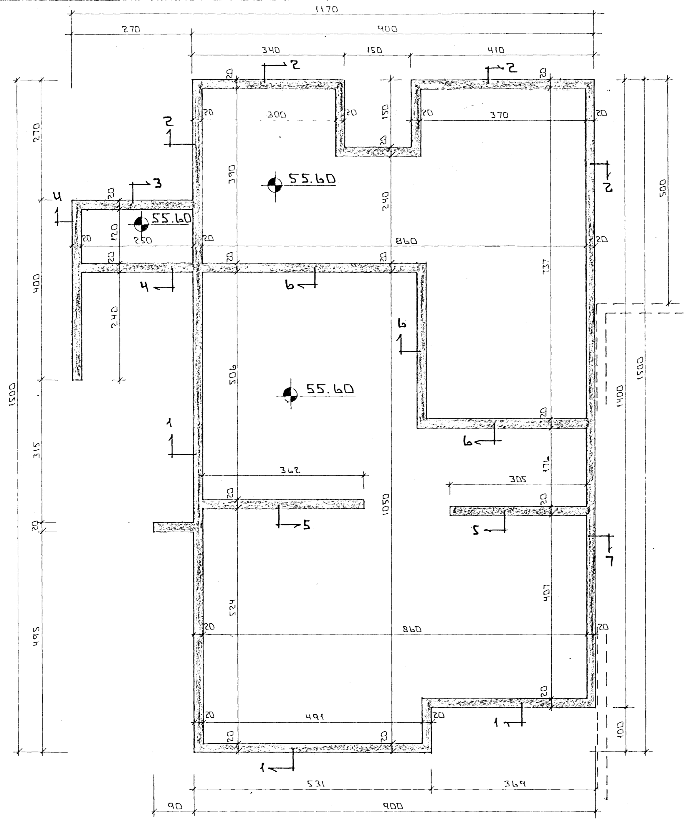
GRUNNMÝND 1:50
