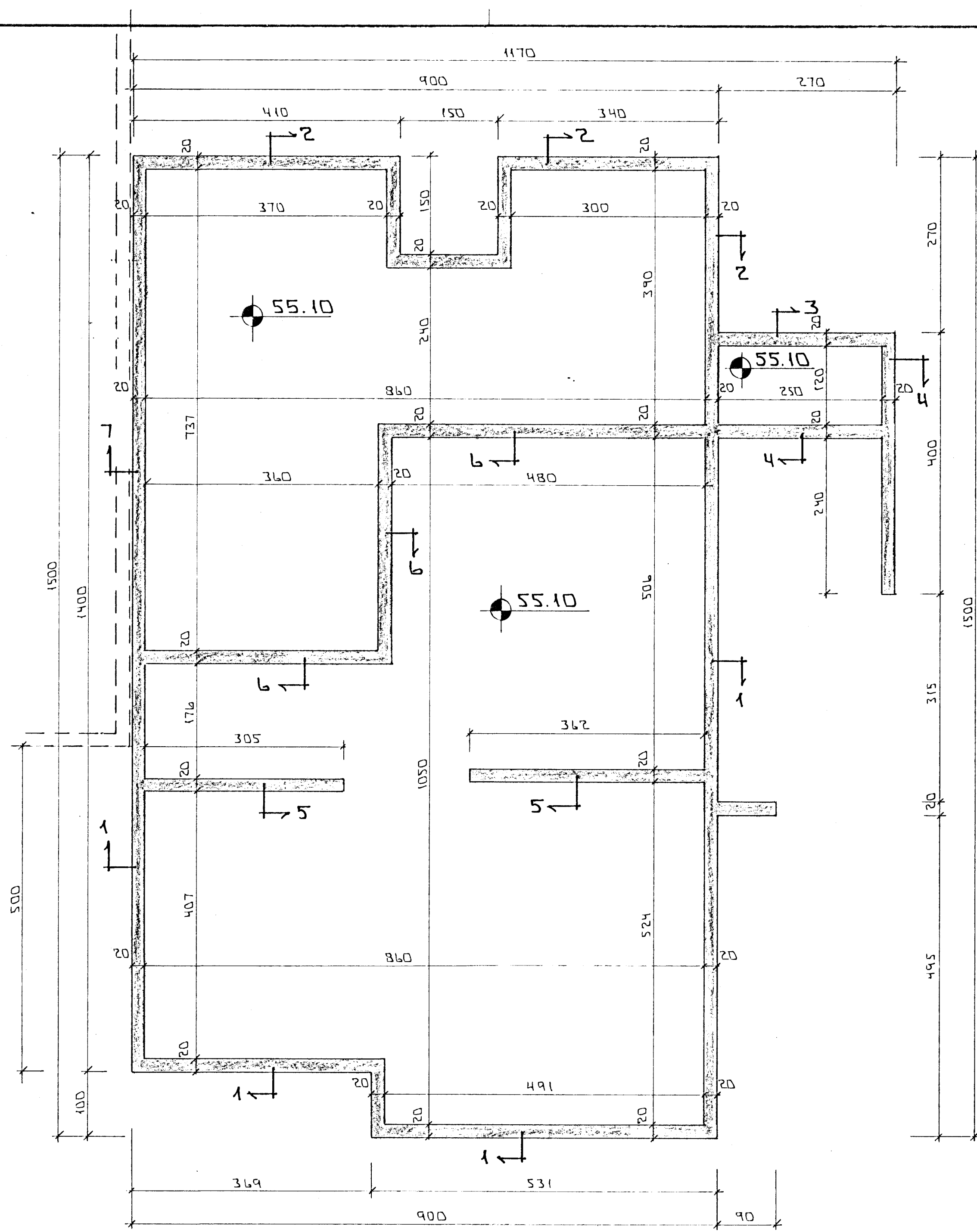
GRUNNMÝND 1 : 50
