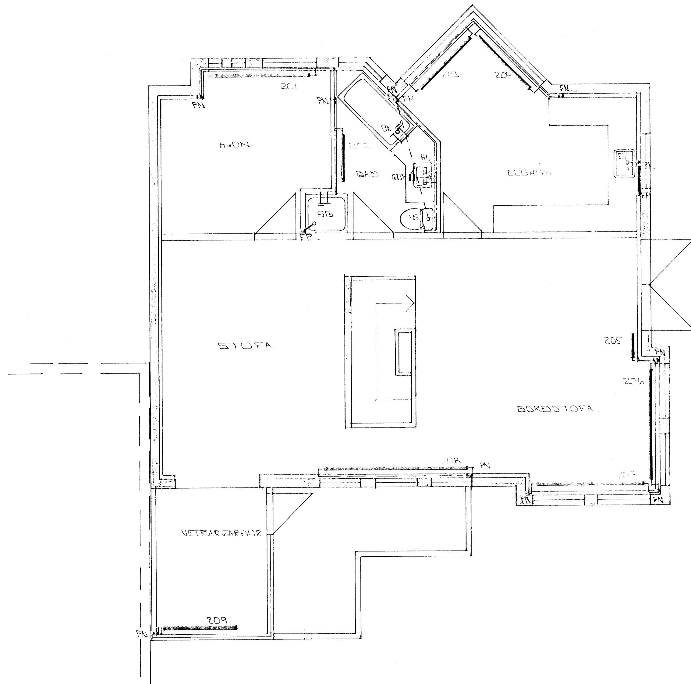
GRUNNMÝND 2. HÆÐ 1:50
