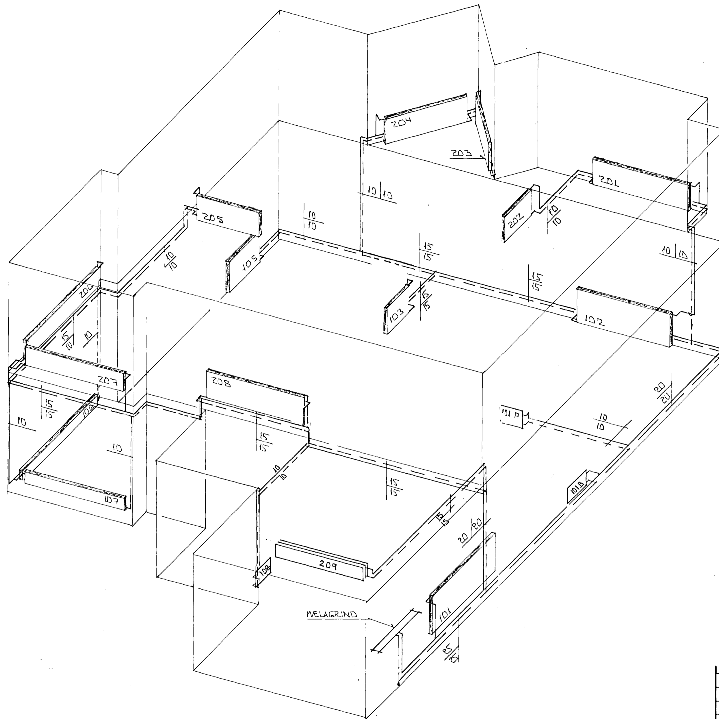
RÚMMYND HITALAGNA 1:50
