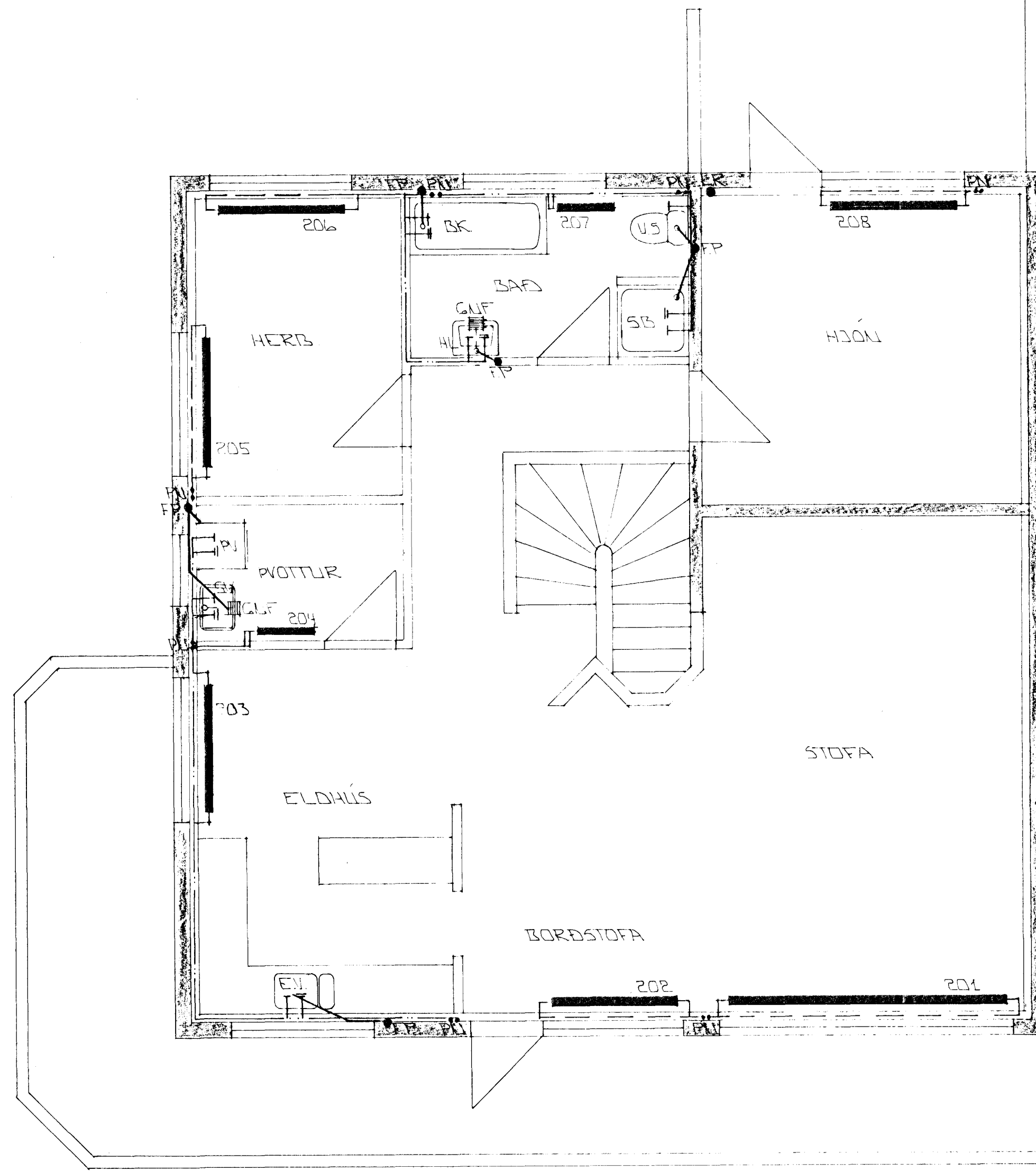
GRUNNMÝND 1 : 50
