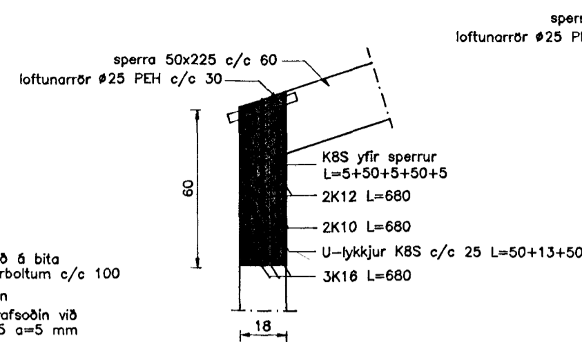
Snið 24-24 Mkv. 1 : 20
