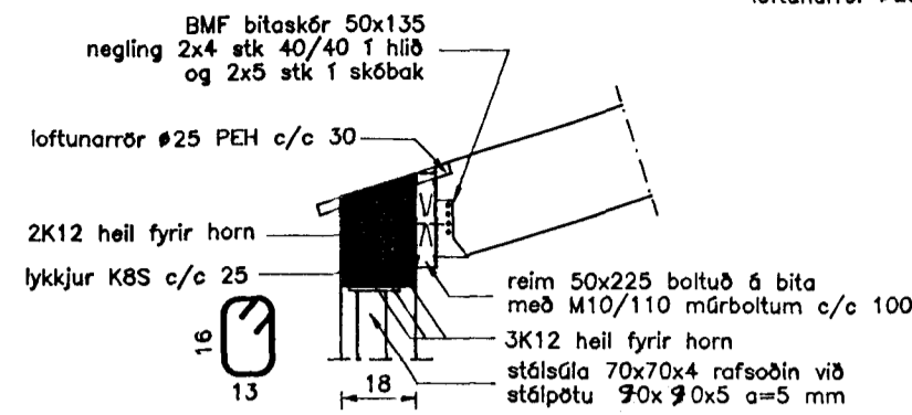
Snið 23-23 Mkv. 1 : 20
