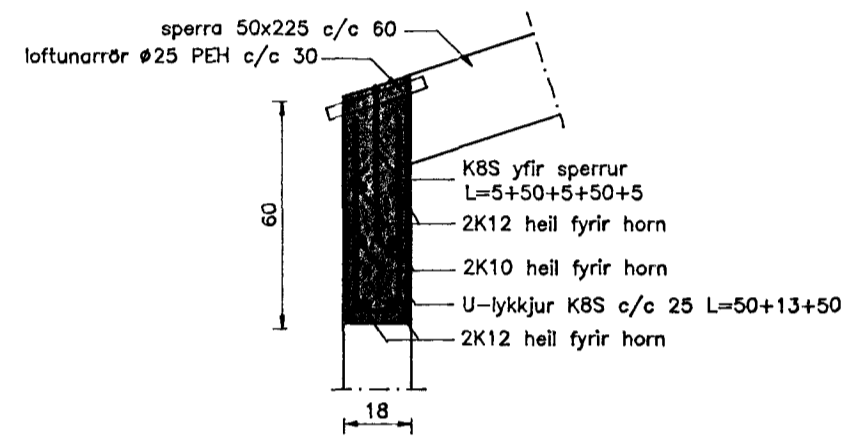
Snið 26-26 Mkv. 1 : 20
