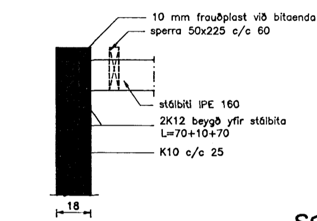
Snið 28-28 Mkv. 1 : 20
