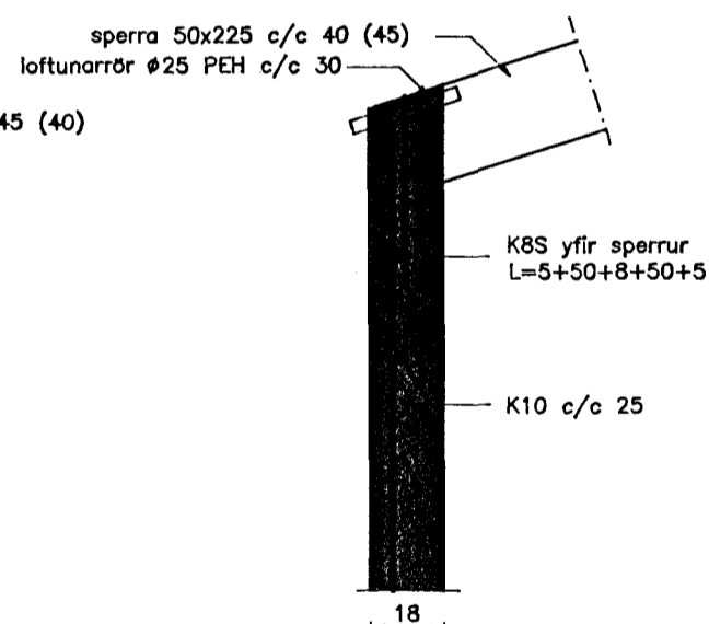
Snið 32-32 Mkv. 1 : 20
