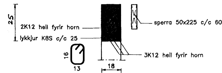
Snið 22a-22a Mkv. 1 : 20
