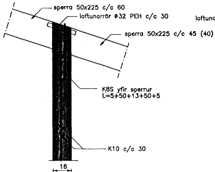
Snið 31-31 Mkv. 1 : 20
