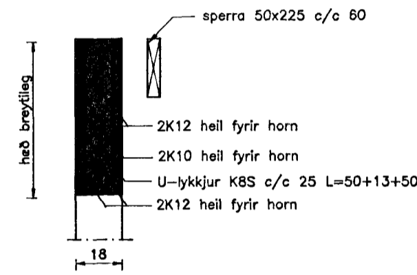
Snið 27-27 Mkv. 1 : 20
