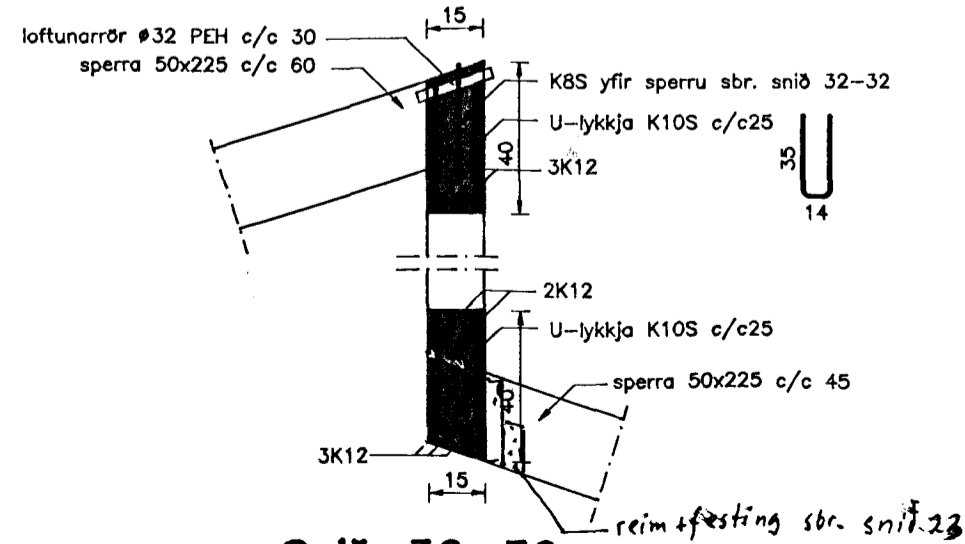
Snið 36-36 Mkv. 1 : 20
