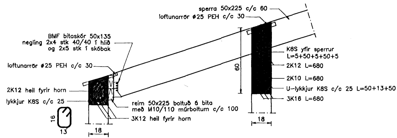
Snið 22-22 Mkv. 1 : 20
