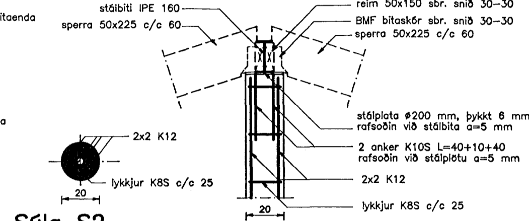
Súla S2 Mkv. 1 : 20
