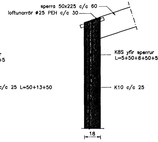
Snið 25-25 Mkv. 1 : 20
