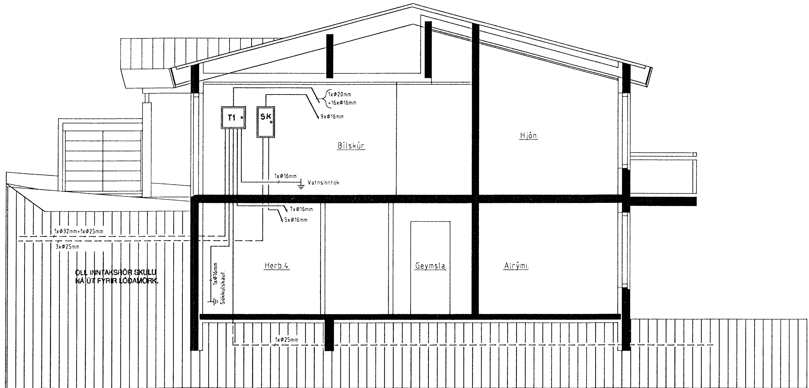
Snið A-A, mælikvarði 1/50.
