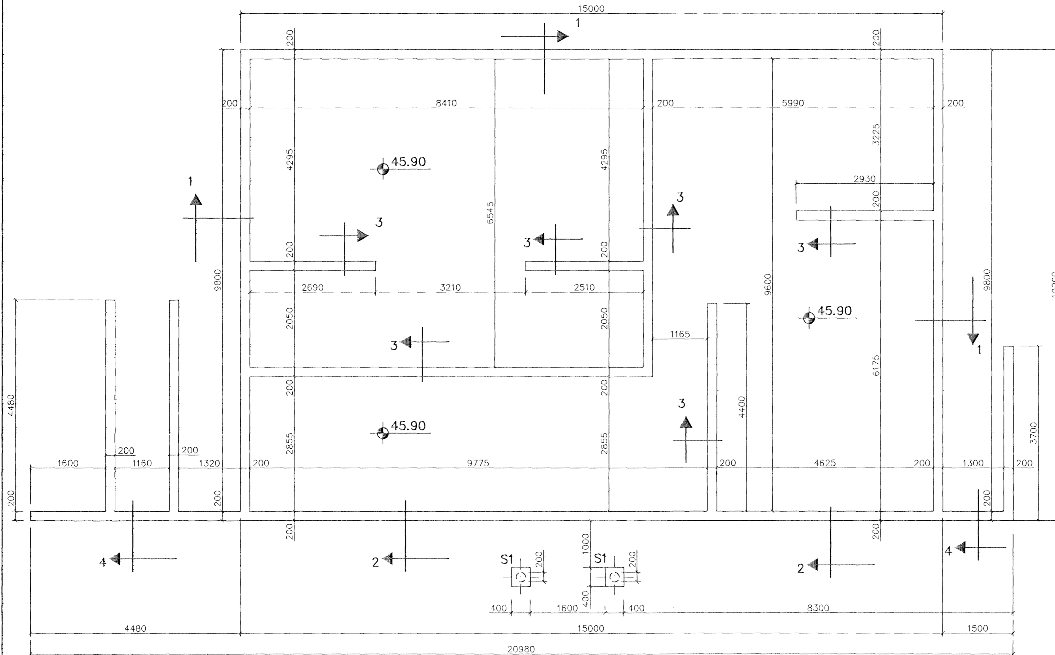
GRUNNMYND 1:50
