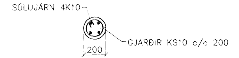
SÚLA S1 1:20
