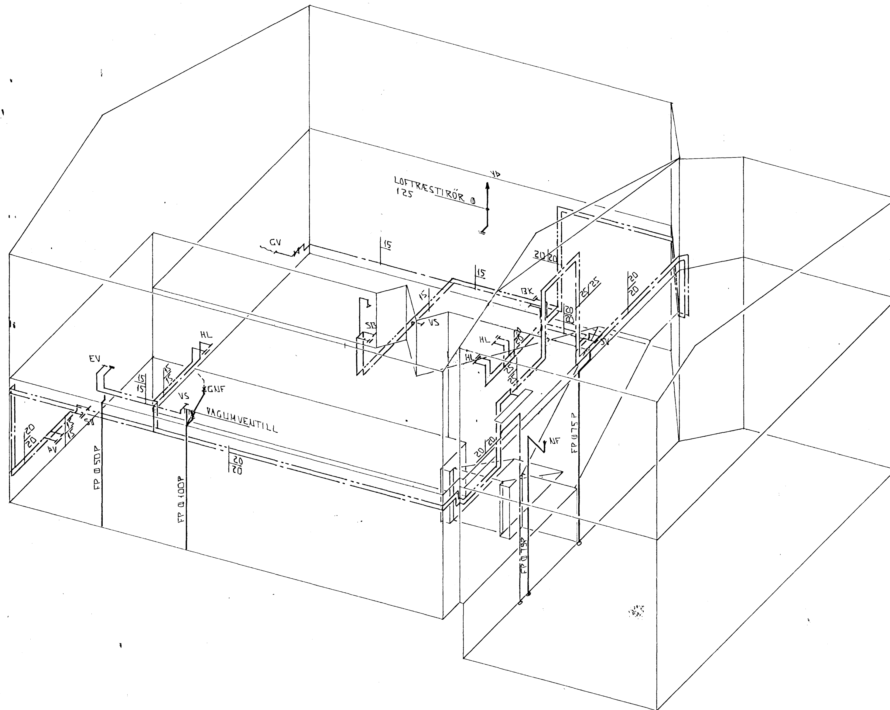
RÚMMYND - VATNSLAGNA - 1:50
