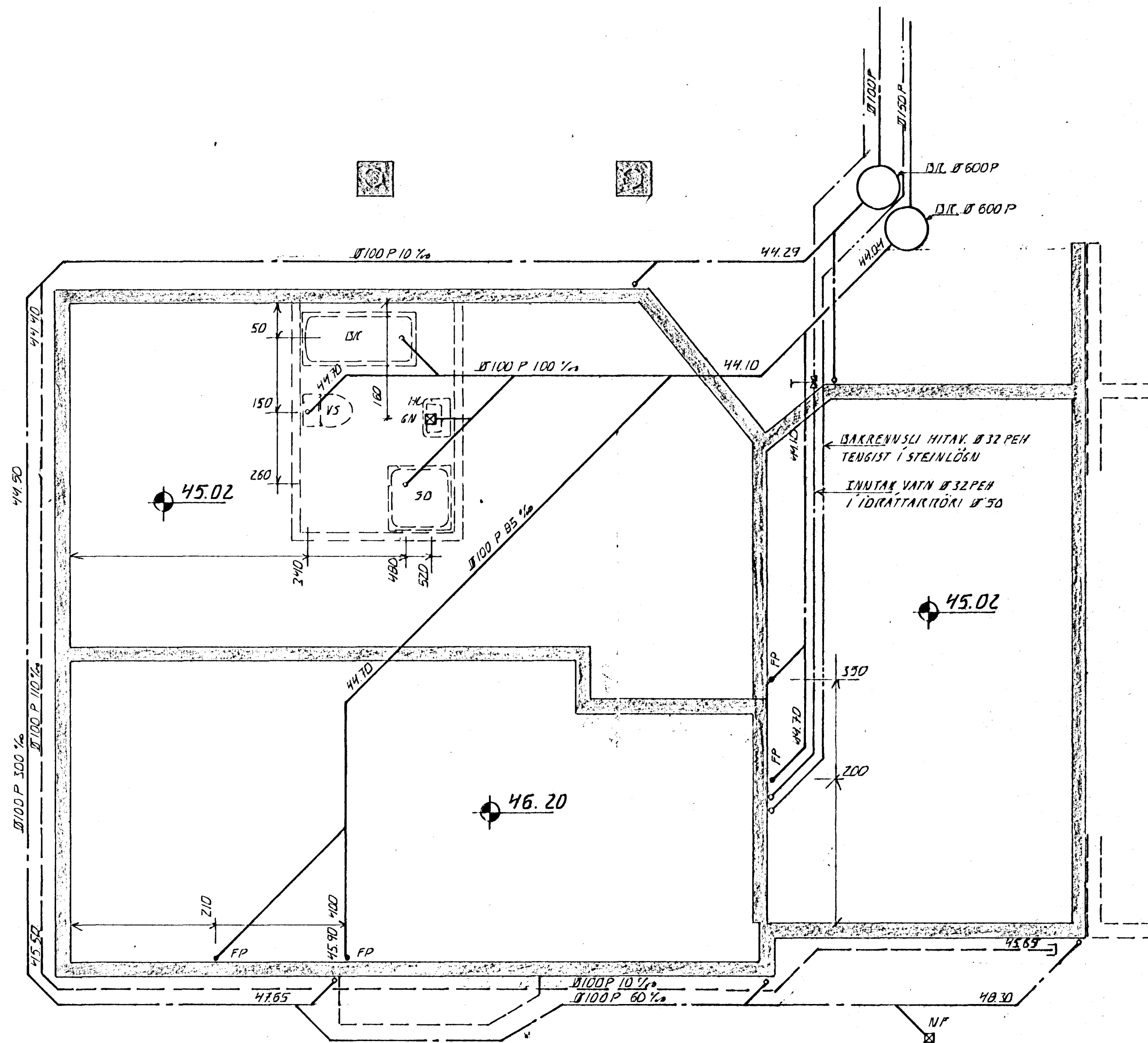
GRUNNMYND, 1:50
