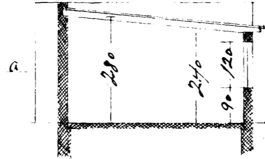
Þverskurður
