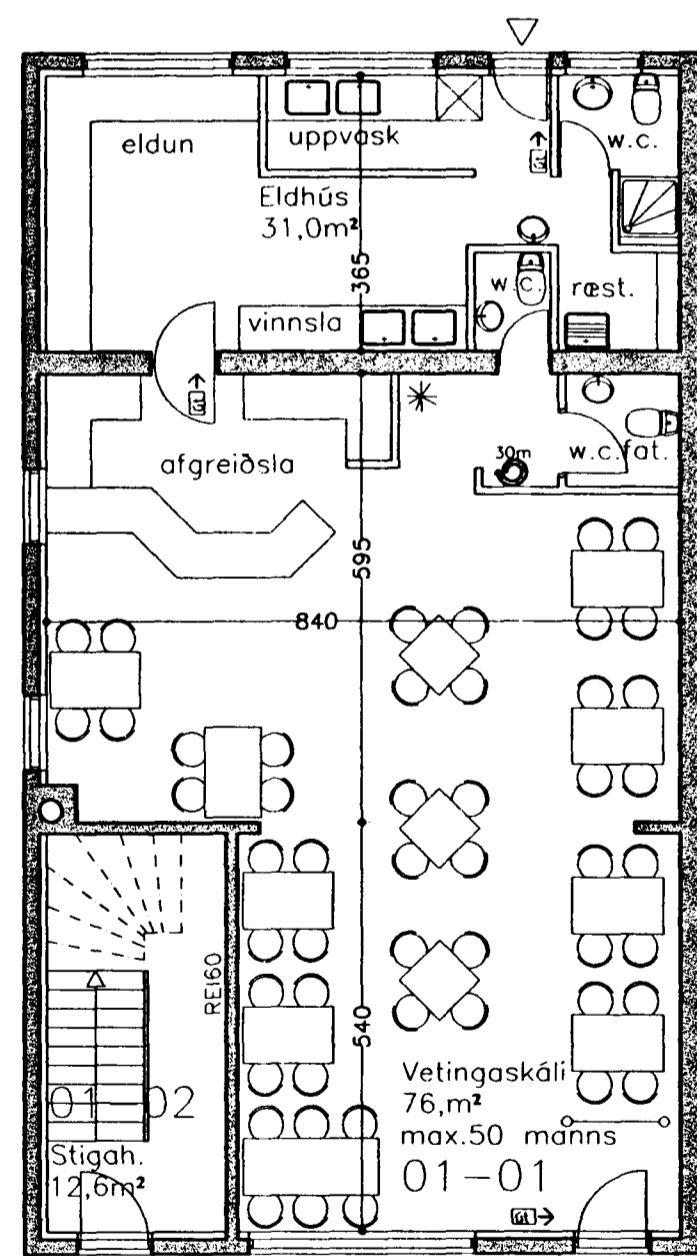
Grunnmynd 1. hæð mkv. 1:100
