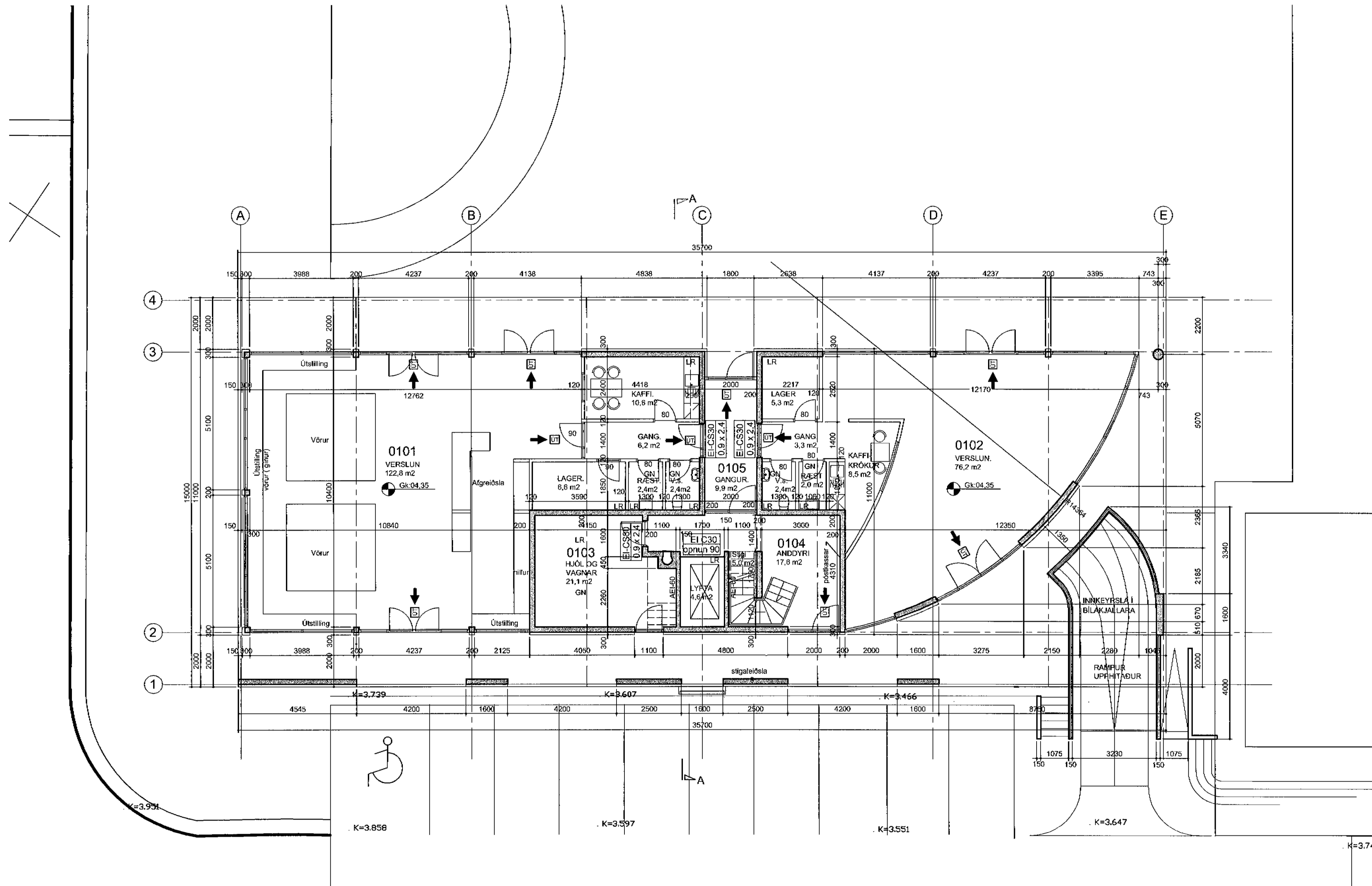
GRUNNMYND 1.HÆÐ MKV 1:100
