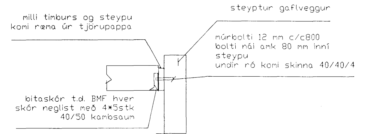
Deili við steyptan gáfl 1/20
