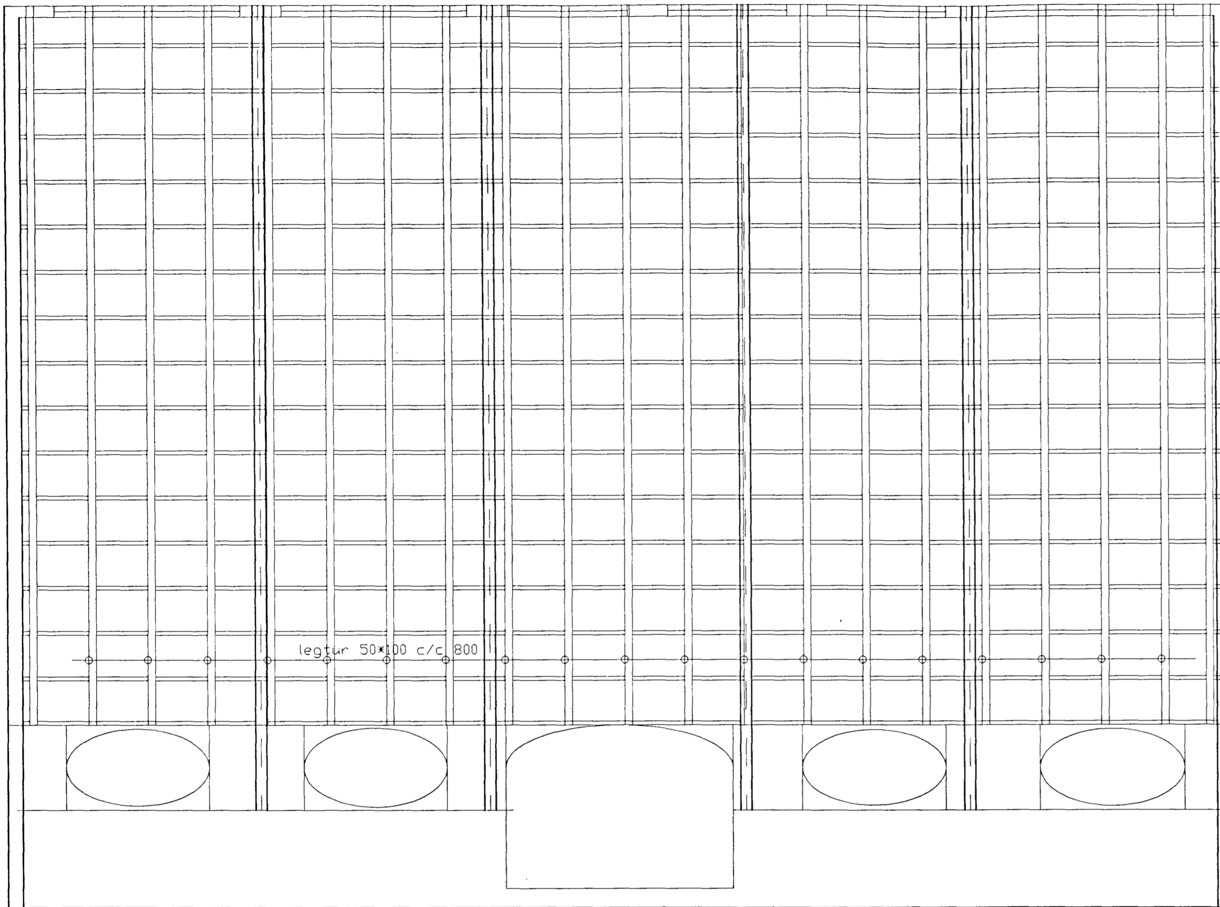
Grunnmynd 5. hæðar 1/50
