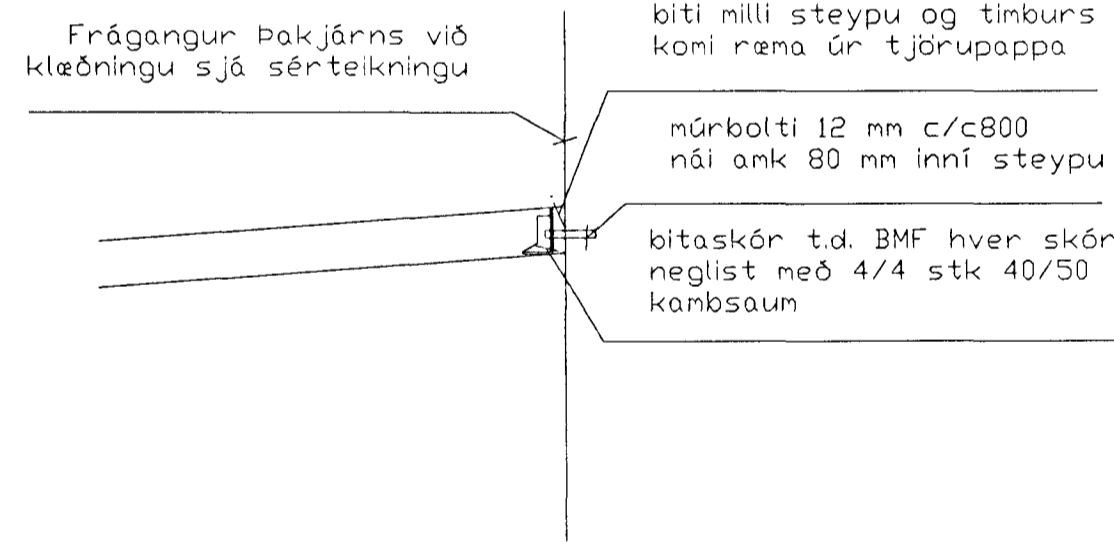
Snið í sperru við hærri vegg 1/20
