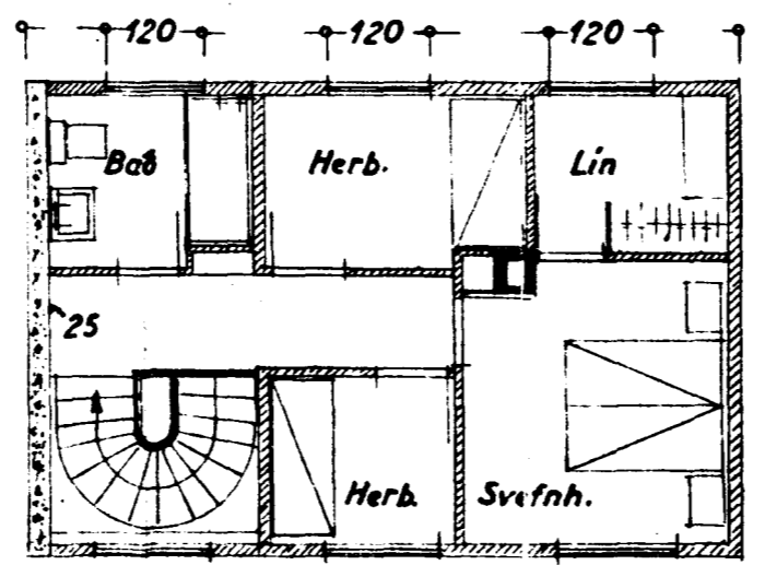
II. hæð
