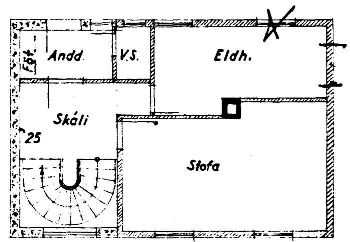
I. hæð
