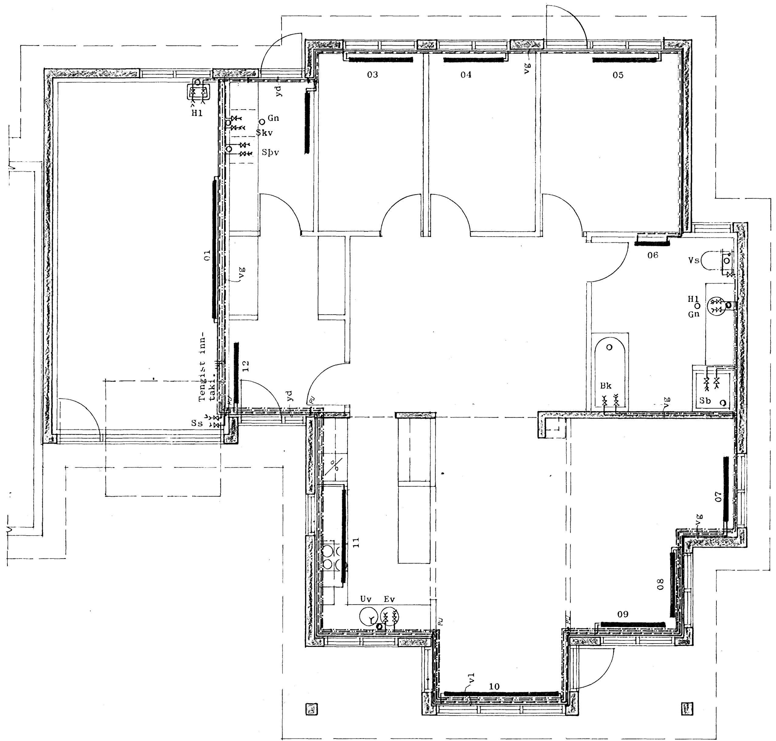
Grunnmynd 1:50
