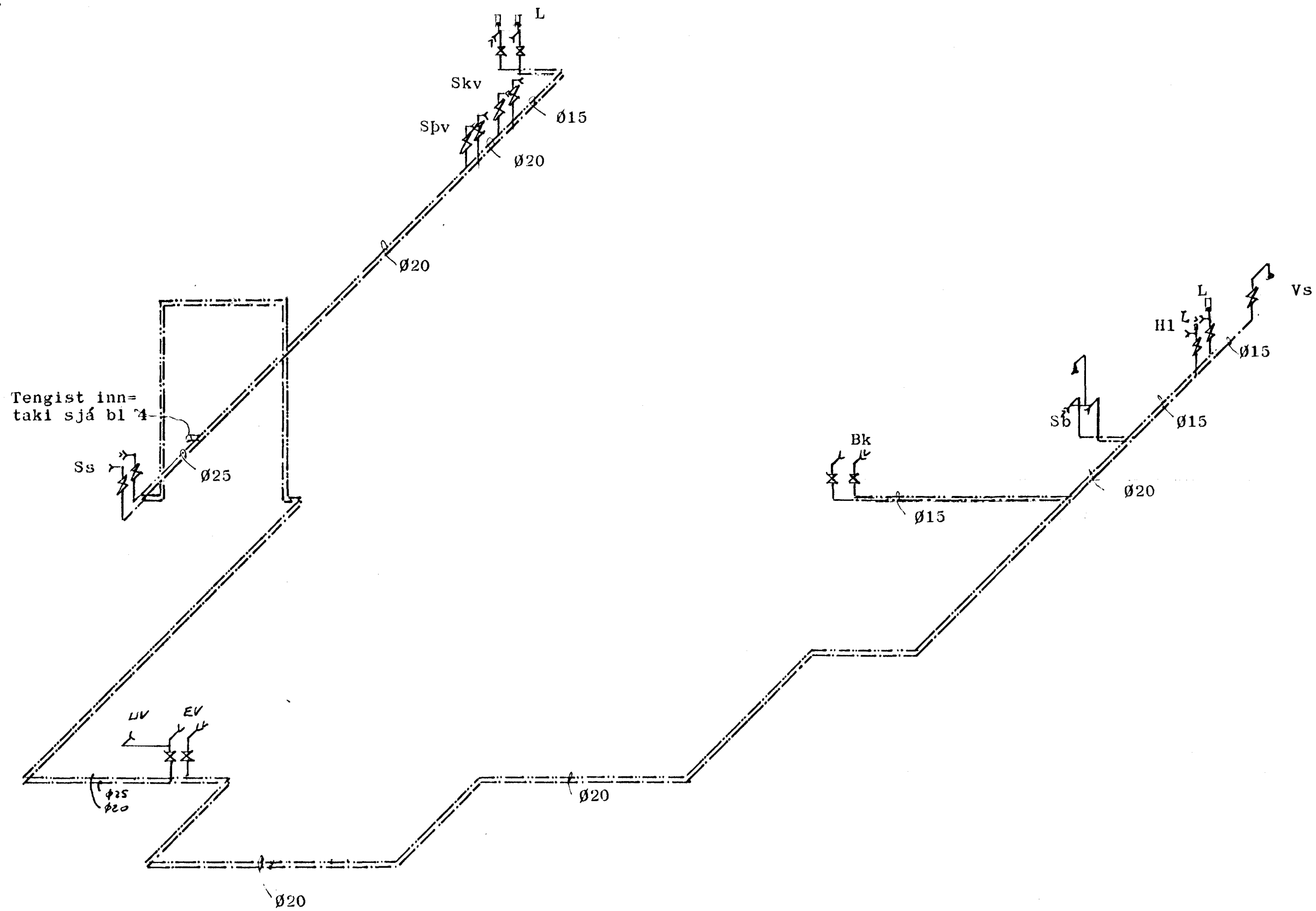
Kerfismynd 1:50
