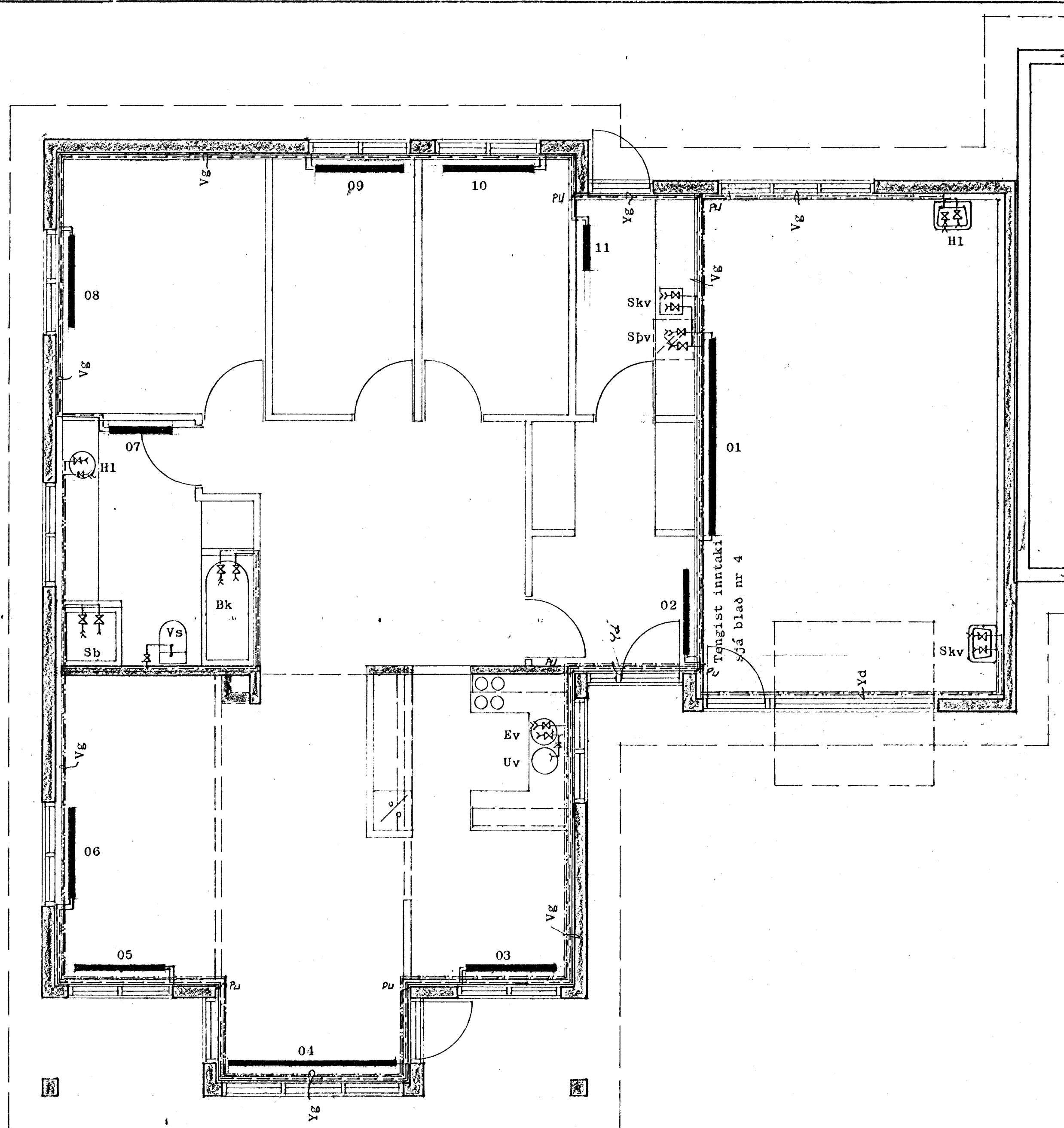
Grunnmynd 1:50
