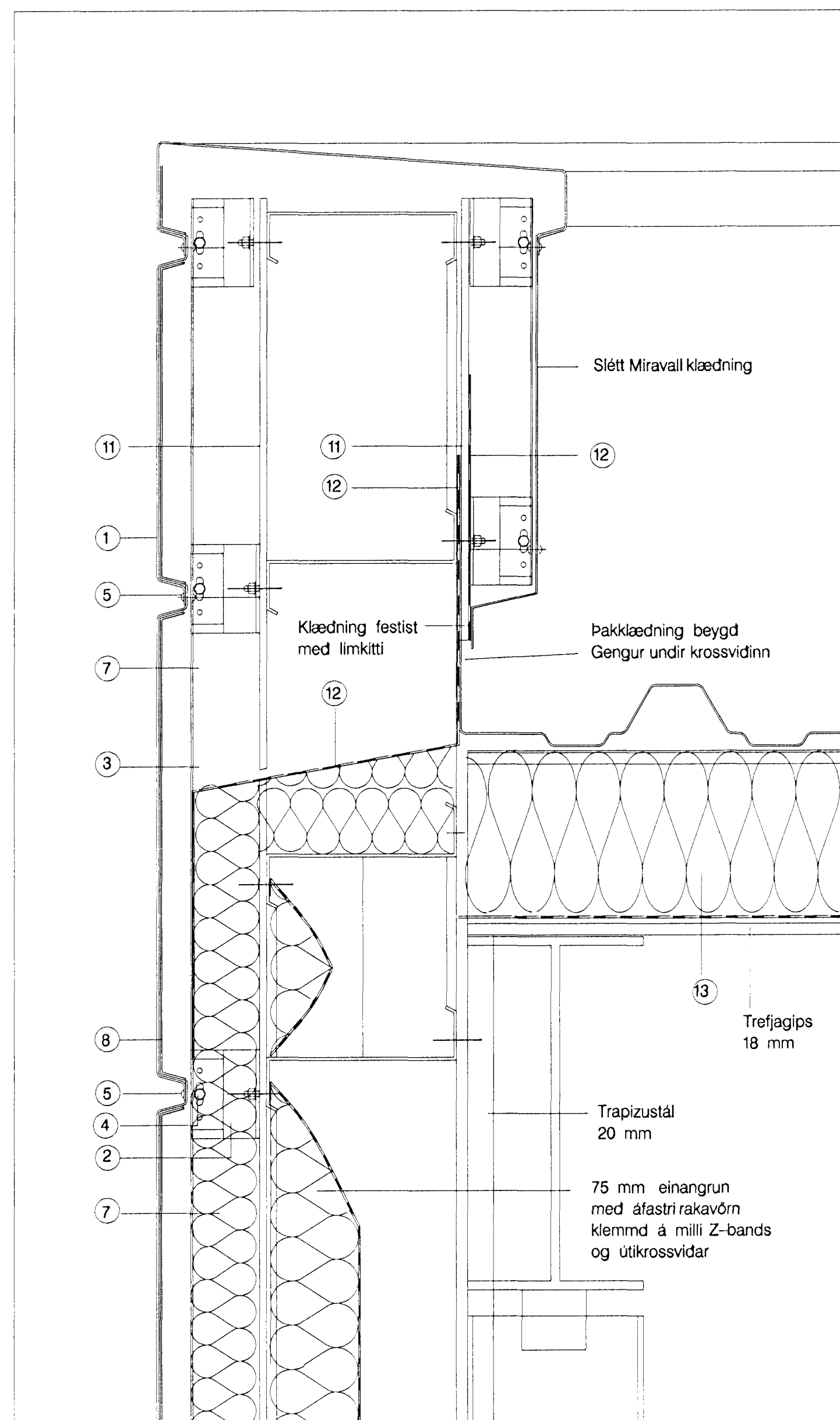
DEILI 8, frágangur þakkanti á göflum
