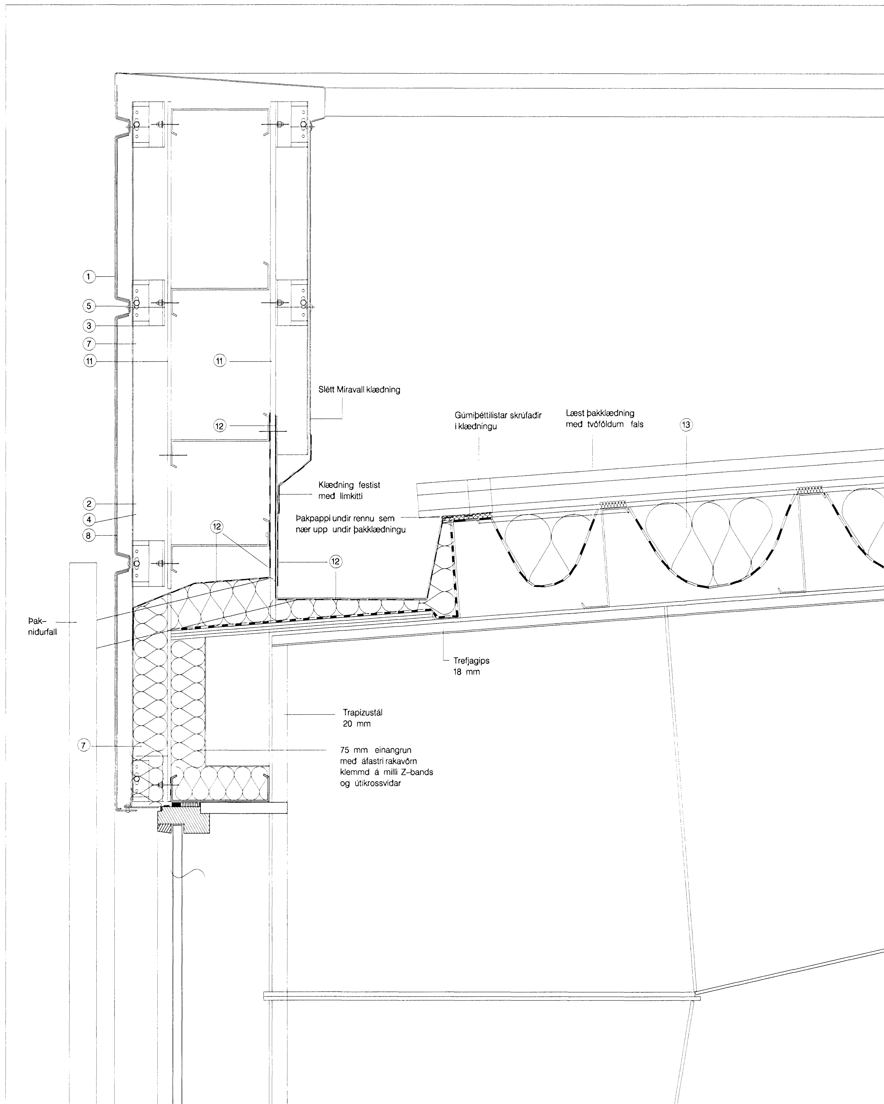
DEILI 7, frágangur þakkants á langhild
