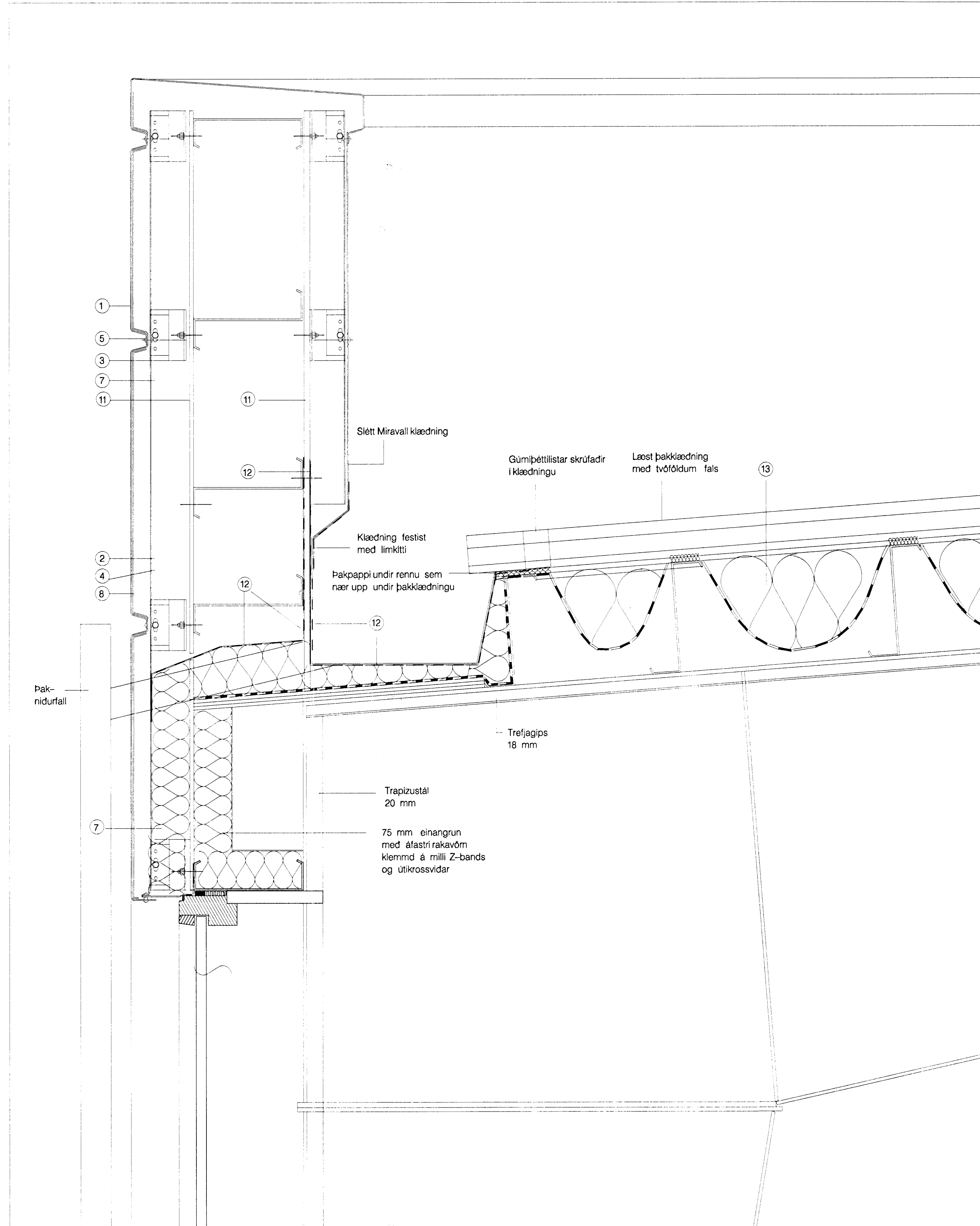
DEILI 7, frágangur þakkants á langhlid
