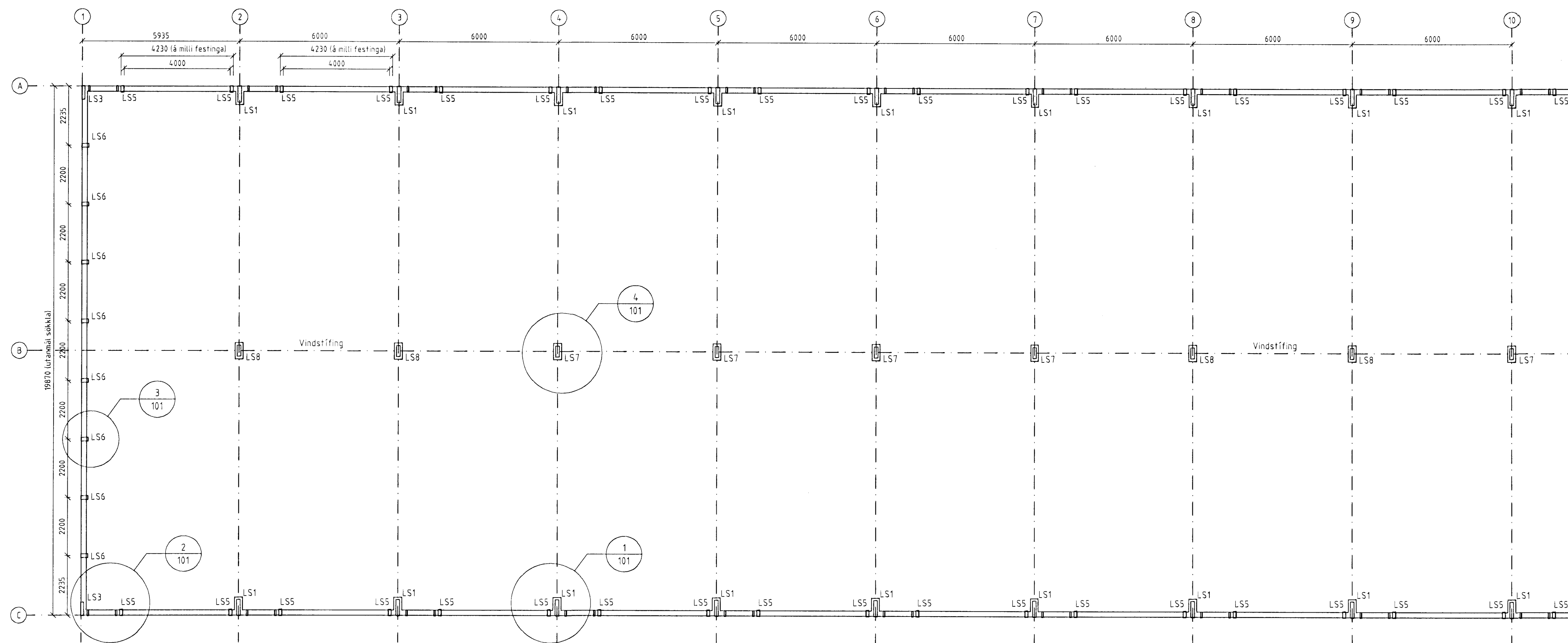
Grunnmynd sökklá Mkv. 1:100
