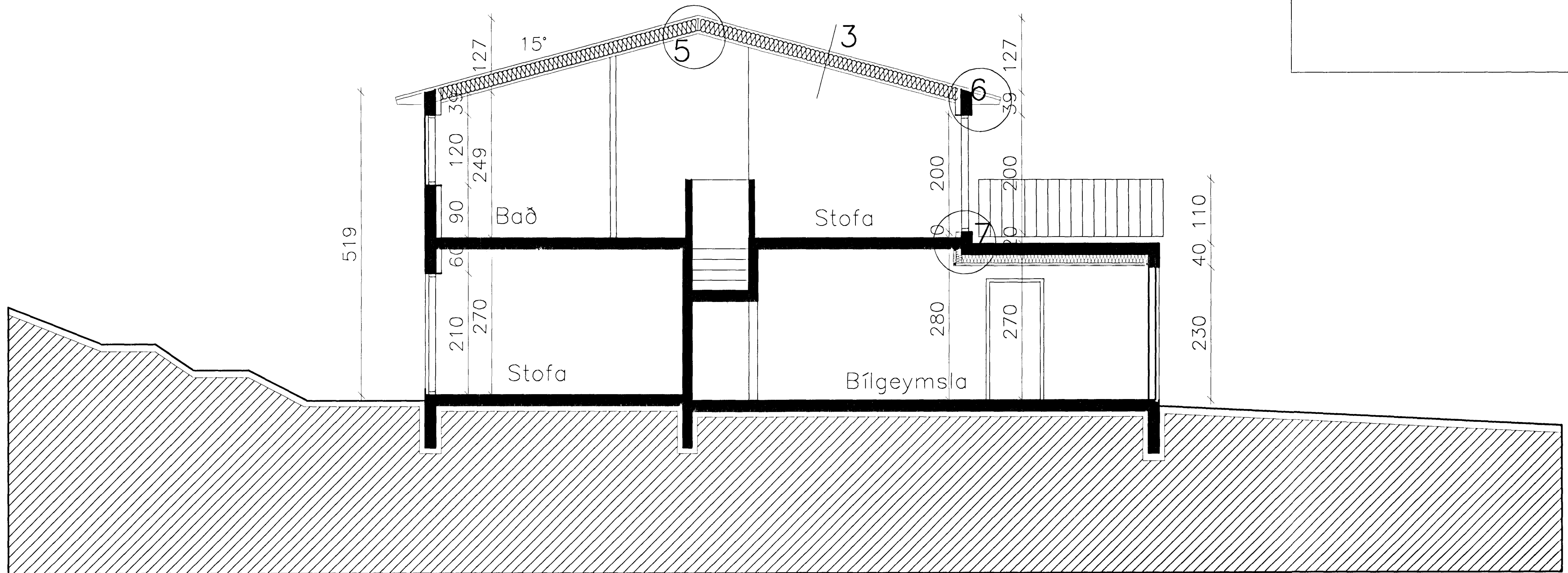
SNEIÐING A-A
