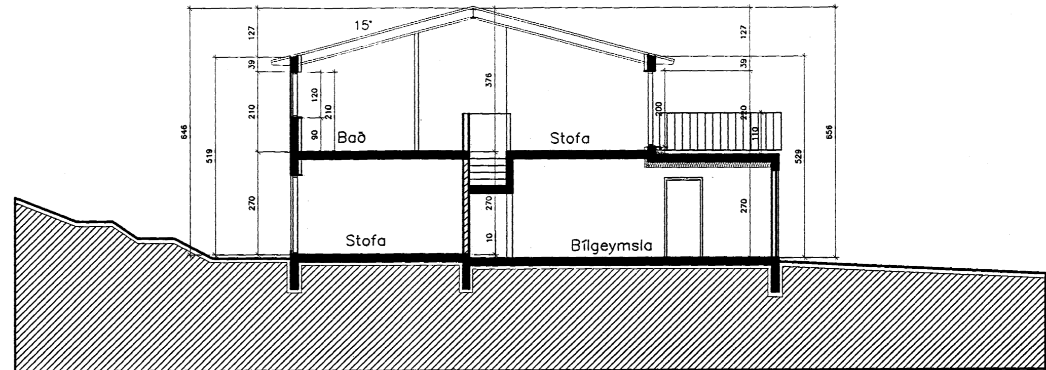
SNEIDING A-A
