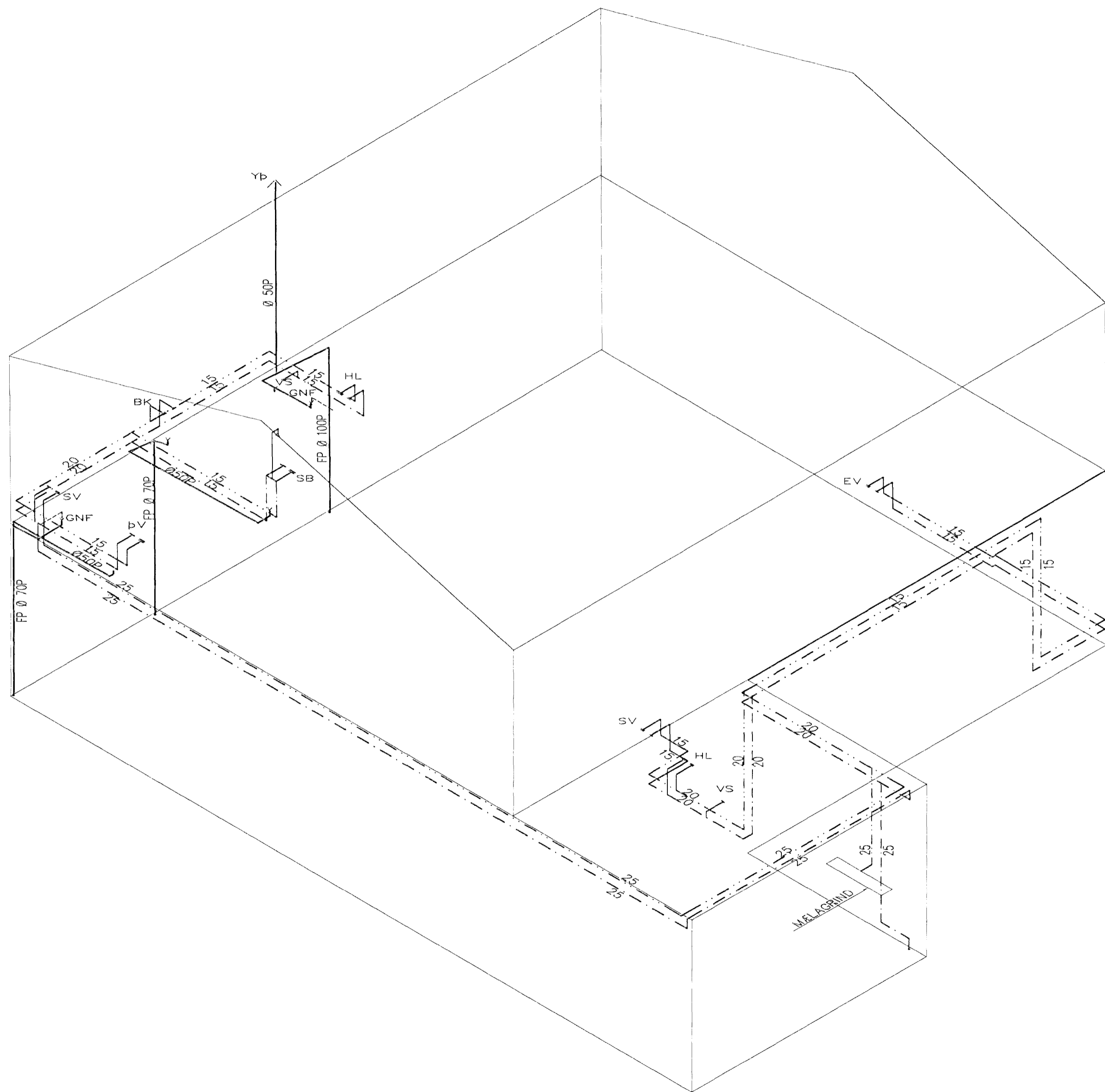
RÜMMYND VATNS OG FRÆRENNSLISLAGNA 1:50
