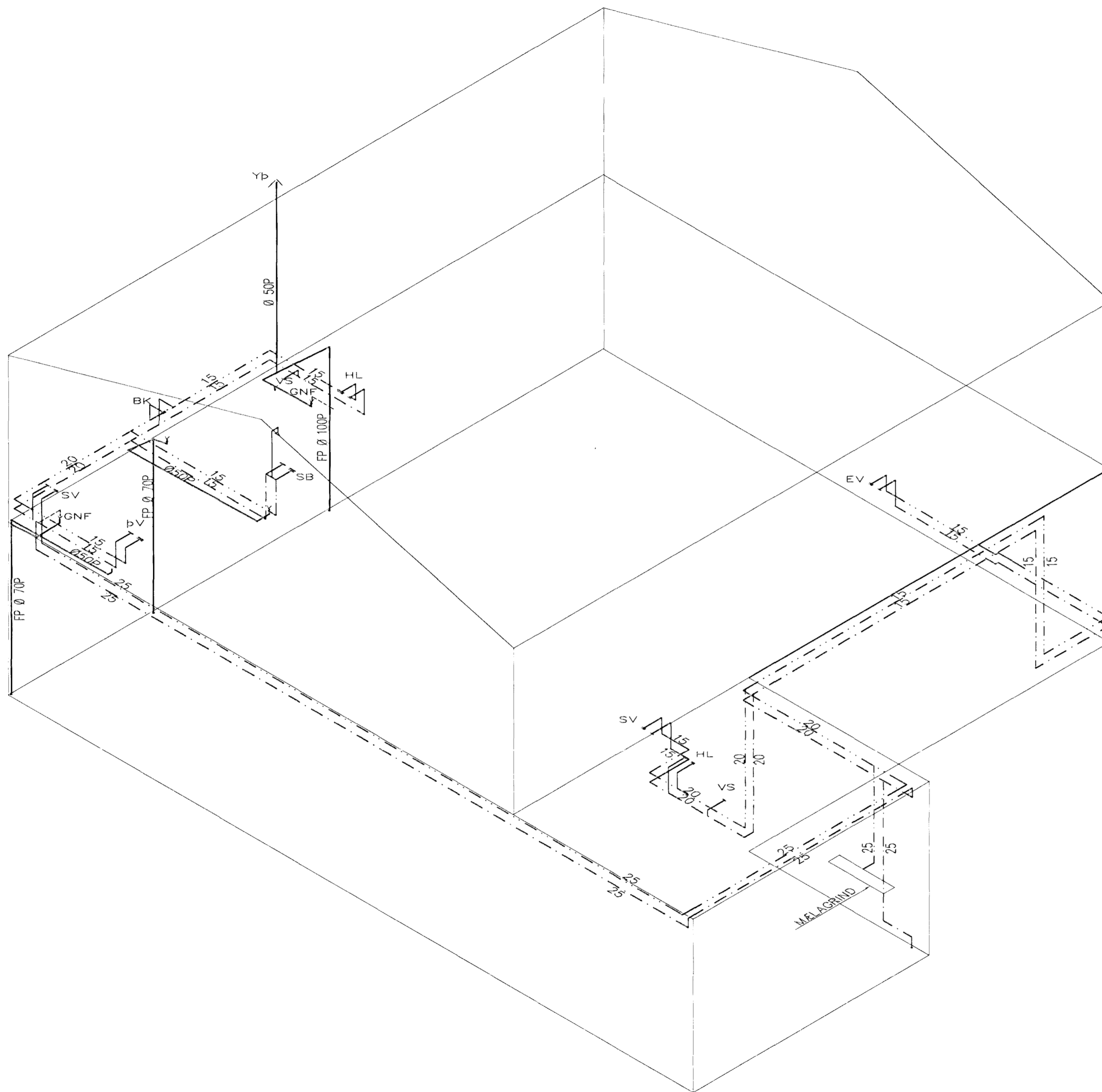
RÚMMYND VATNS OG FRÁRENNISLAGNA 1:50
