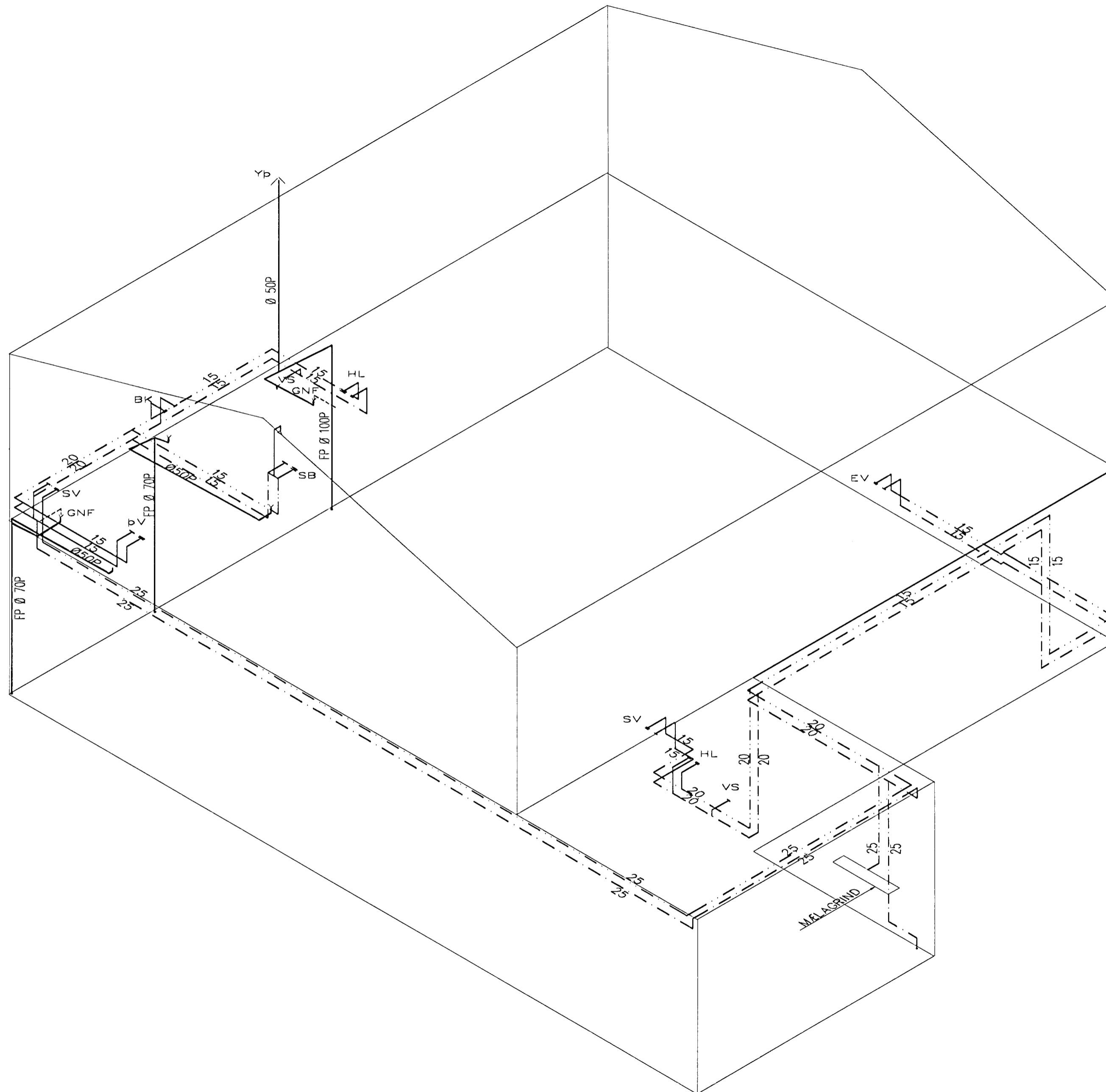
RÚMMYND VATNS OG FRÁRENNSLISLAGNA 1:50
