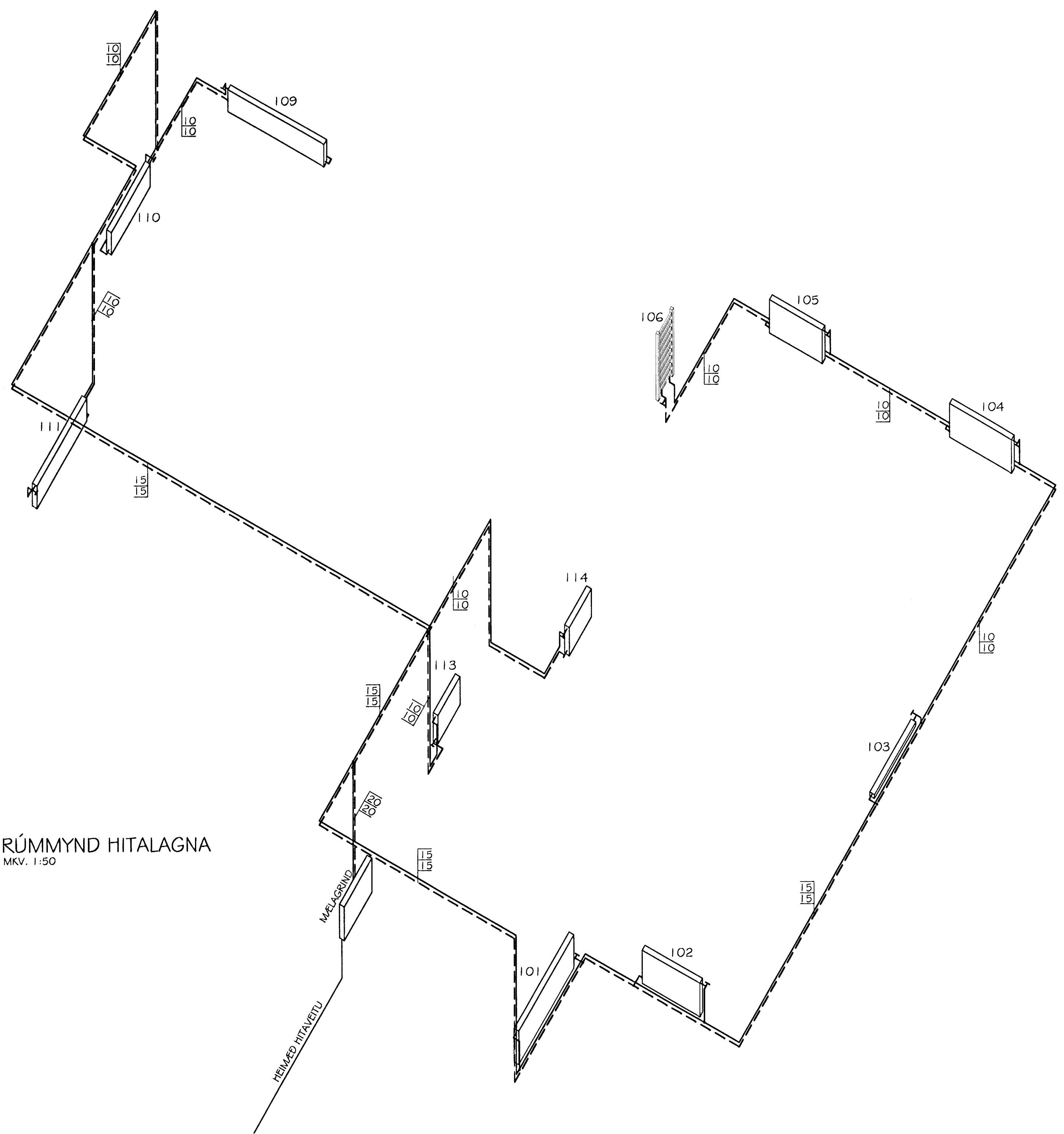
RÚMMYND NEYSLUVATNSLAGNA MKV. 1:50
