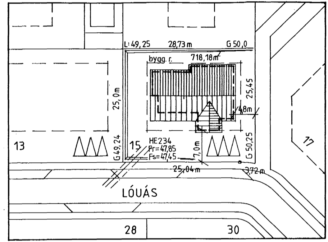
afstöðumynd 1:500
