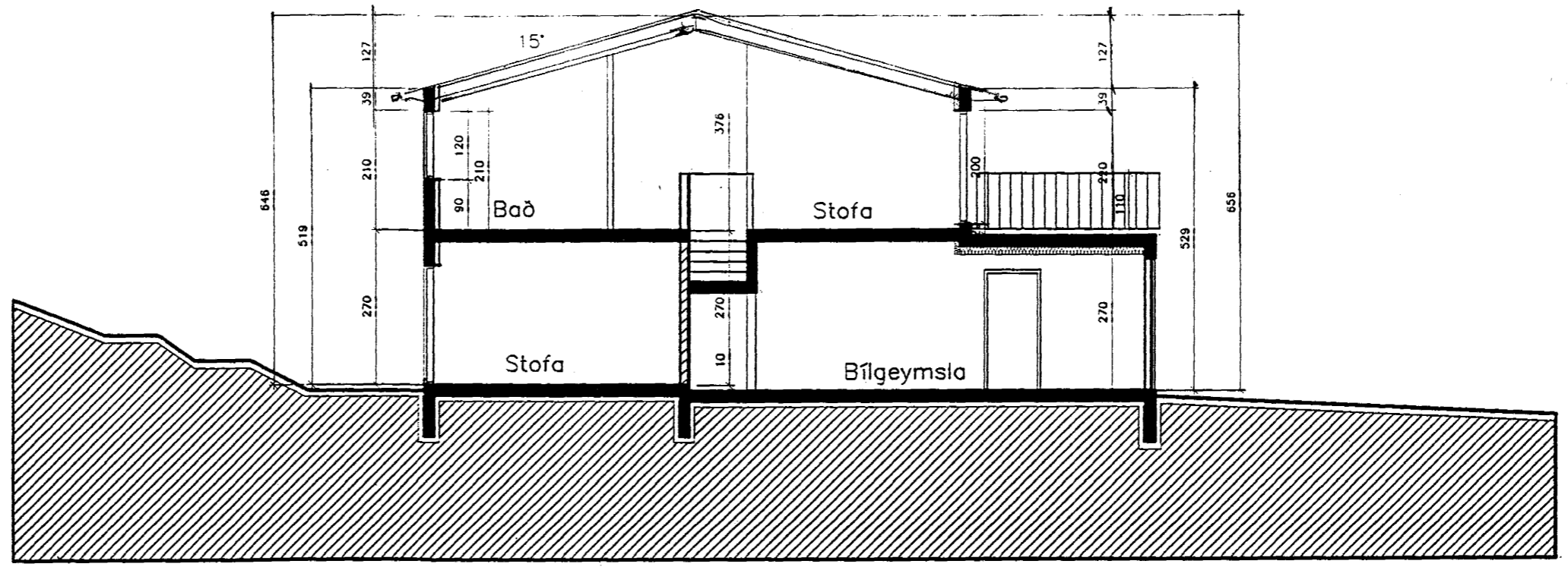
SNEIDING A-A
