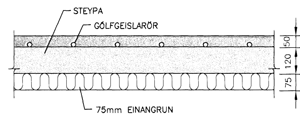
SNID Í GÖLFGEISLALÖGN 1:20
