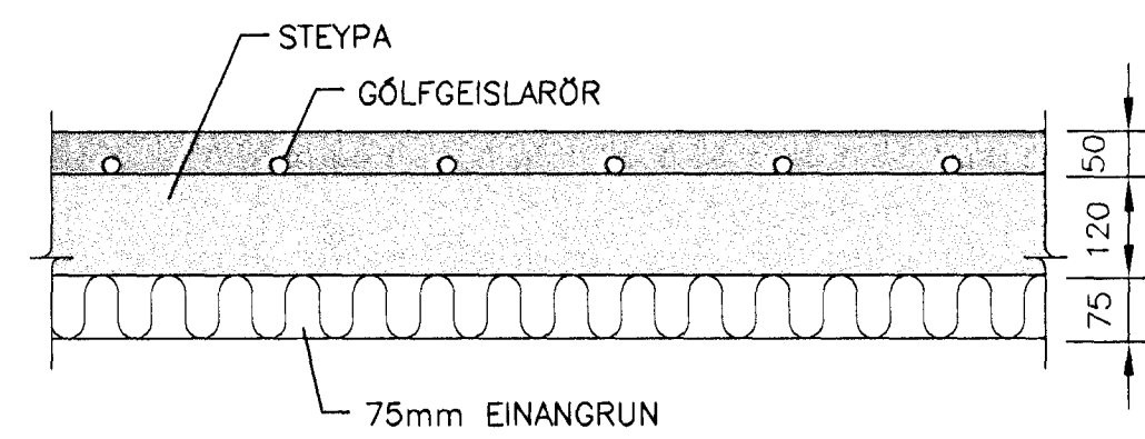
SNID / GÓLFGEISLALÖGN 1:20
