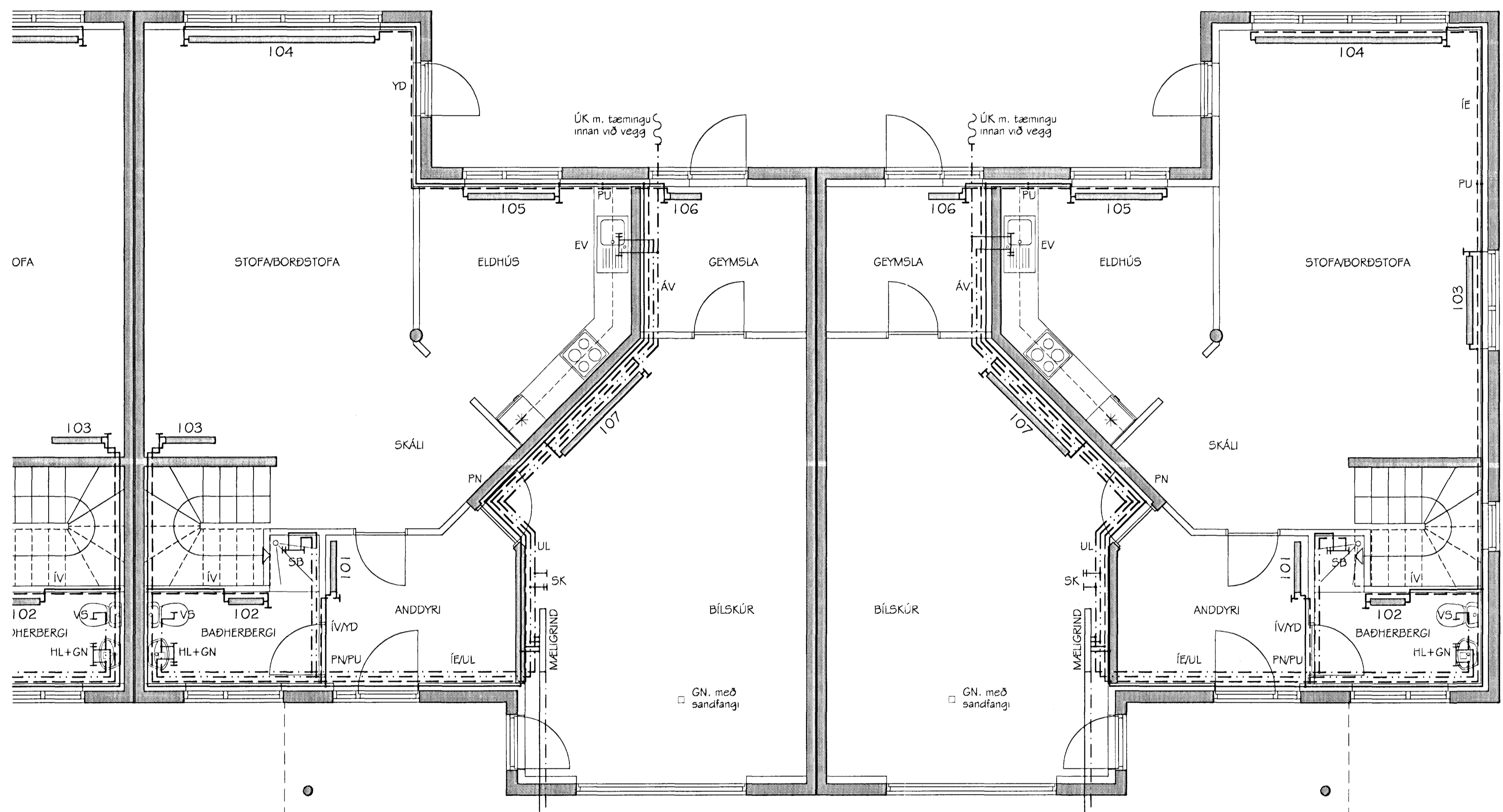
LÓUÁS 18 OG 20 HITA- OG NEYSLUVATNSLAGNIR GRUNNMÝND NEDRI HÆÐAR MKV. 1:50
