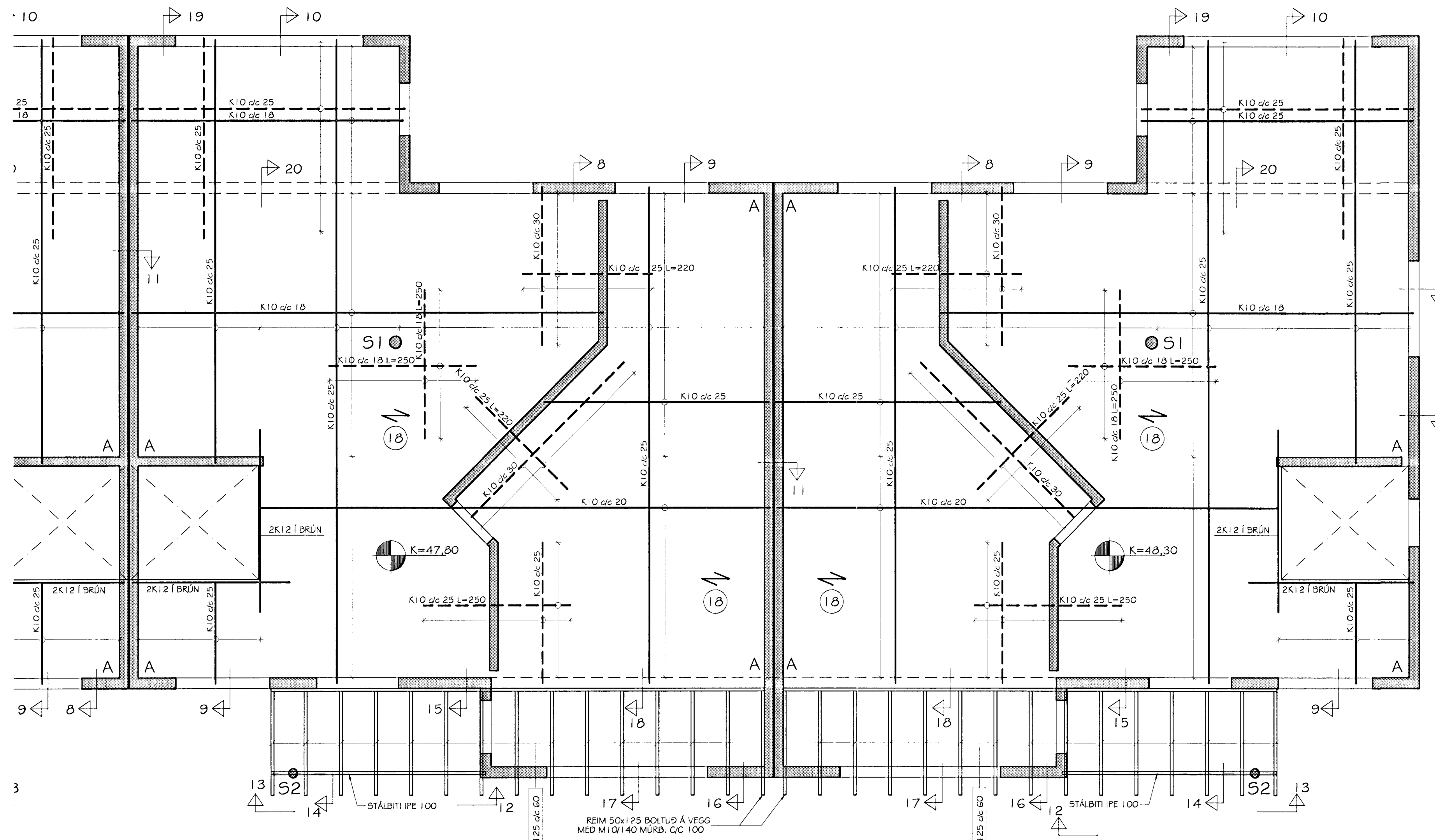
LÓUÁS 18 OG 20 JÁRN Í PLÖTU YFIR 1. HÆÐ OG GRUNNMYND ÞAKVIÐA MKV. 1:50
