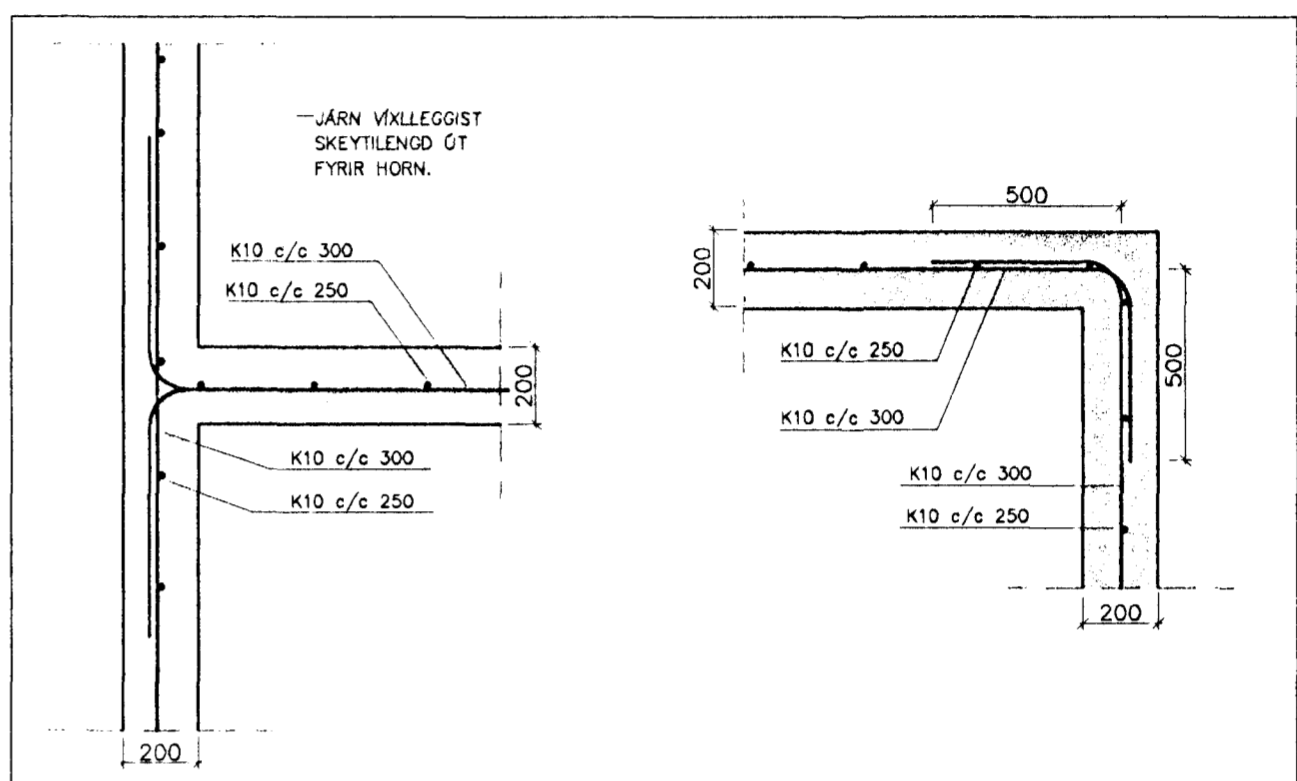
LÁRÉTT SNID Í SÖKKULVEGG Mkv. 1:20
