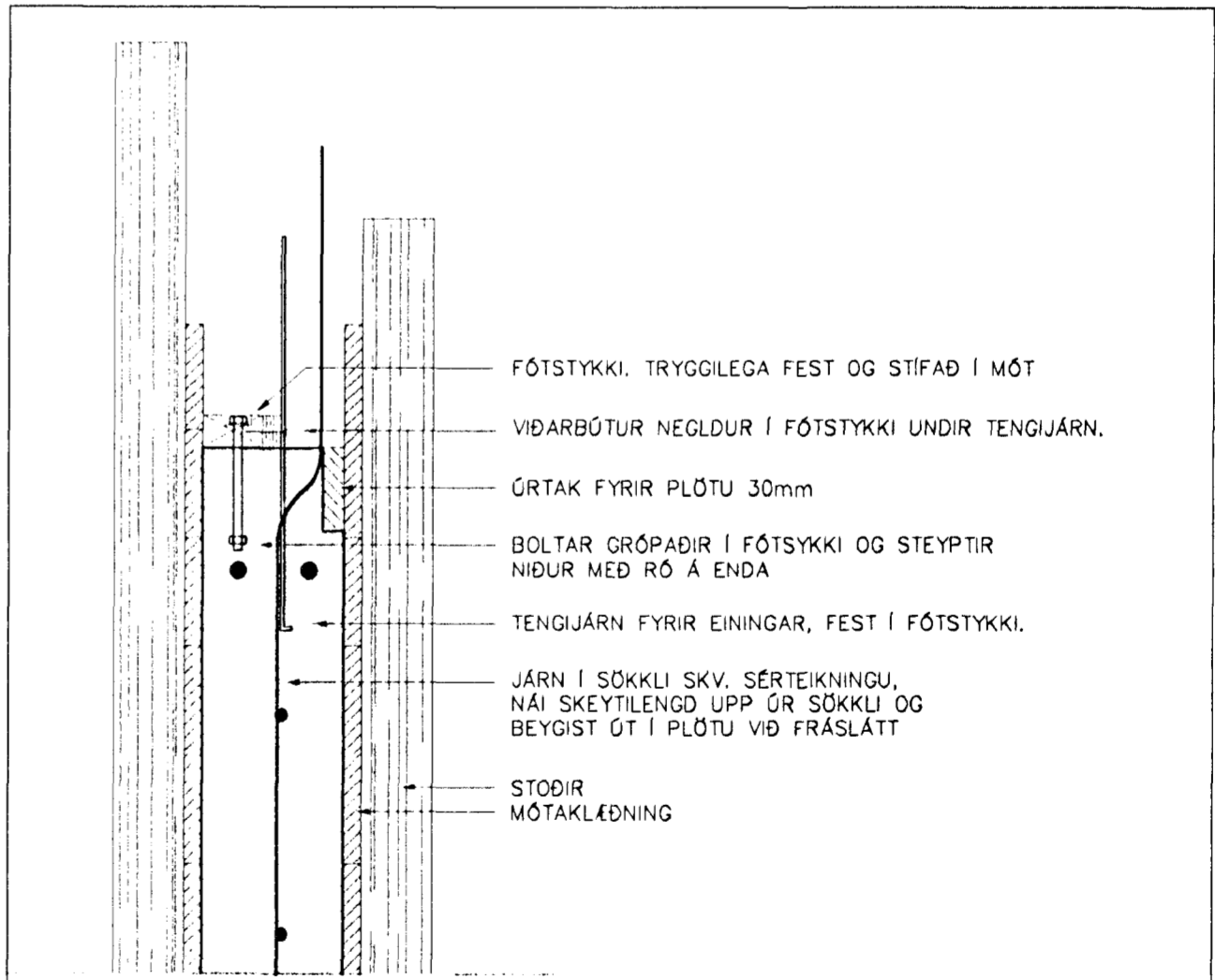
UPPSLÁTTUR Mkv. 1:10
