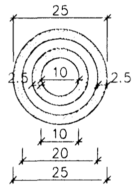
ÞVERSKURÐUR Í RÖR Mkv. 1:1
