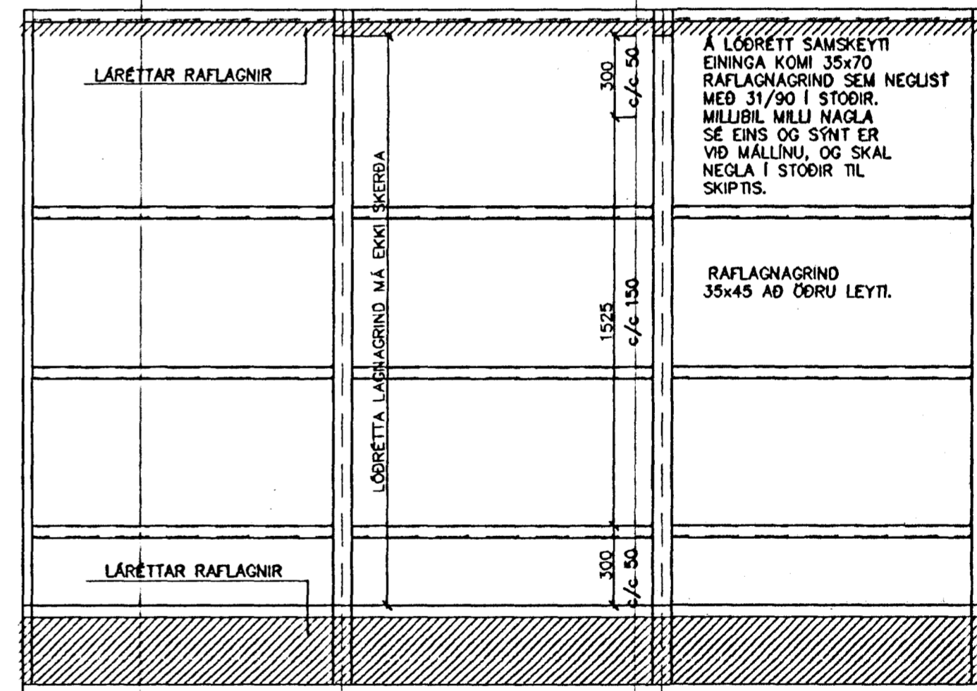
FRÁGANGUR RAFLAGNAGRINDAR Mkv. 1:20
