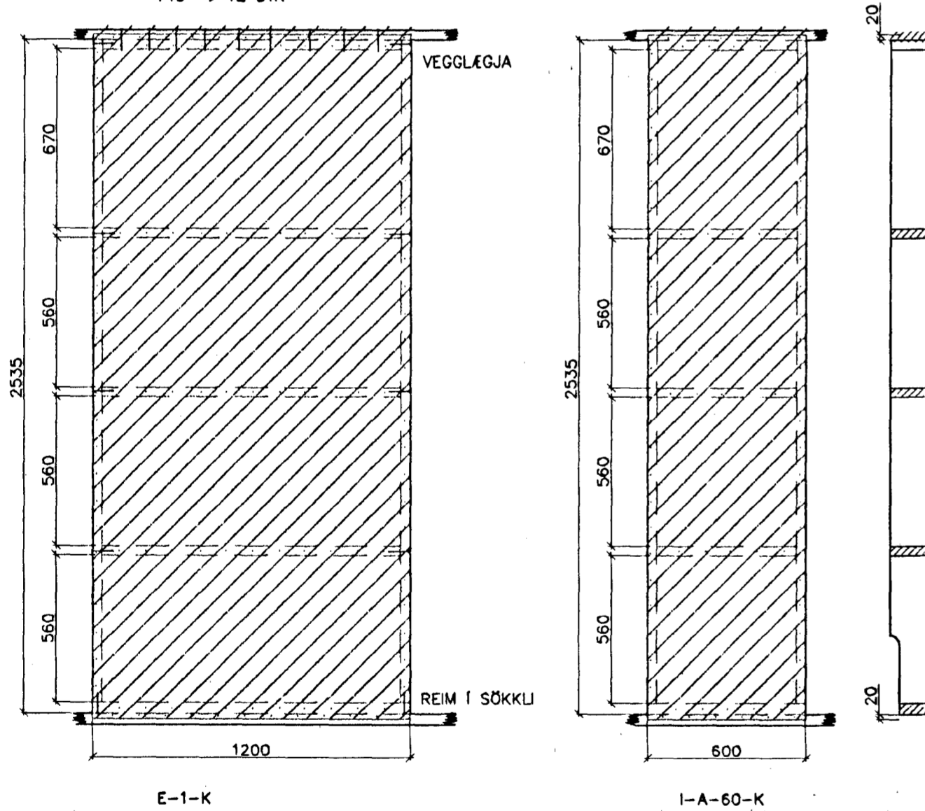
KRÖSSVIÐARSTÍFINGAR Mkv. 1:20
