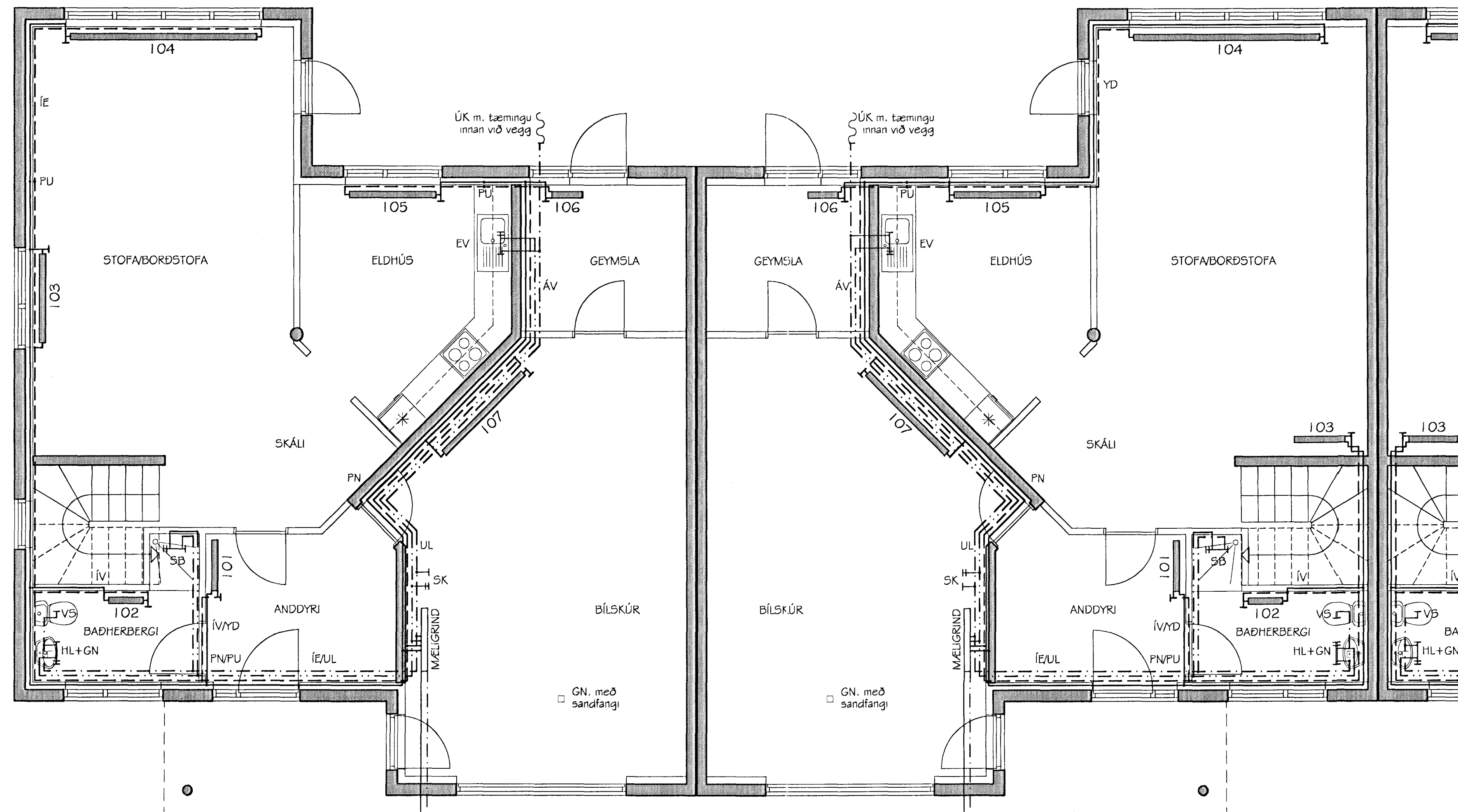
LÓUÁS 22 OG 24 HITA- OG NEYSLUVATNSLAGNIR GRUNNMYND NEDRI HÆÐAR MKV. 1:50
