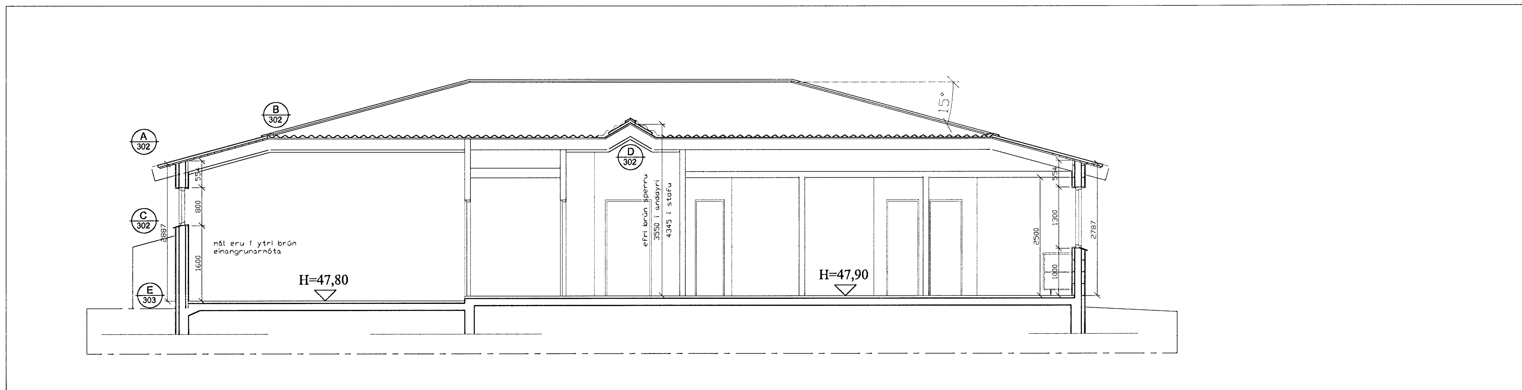
sneiðing a-a, 1:50
