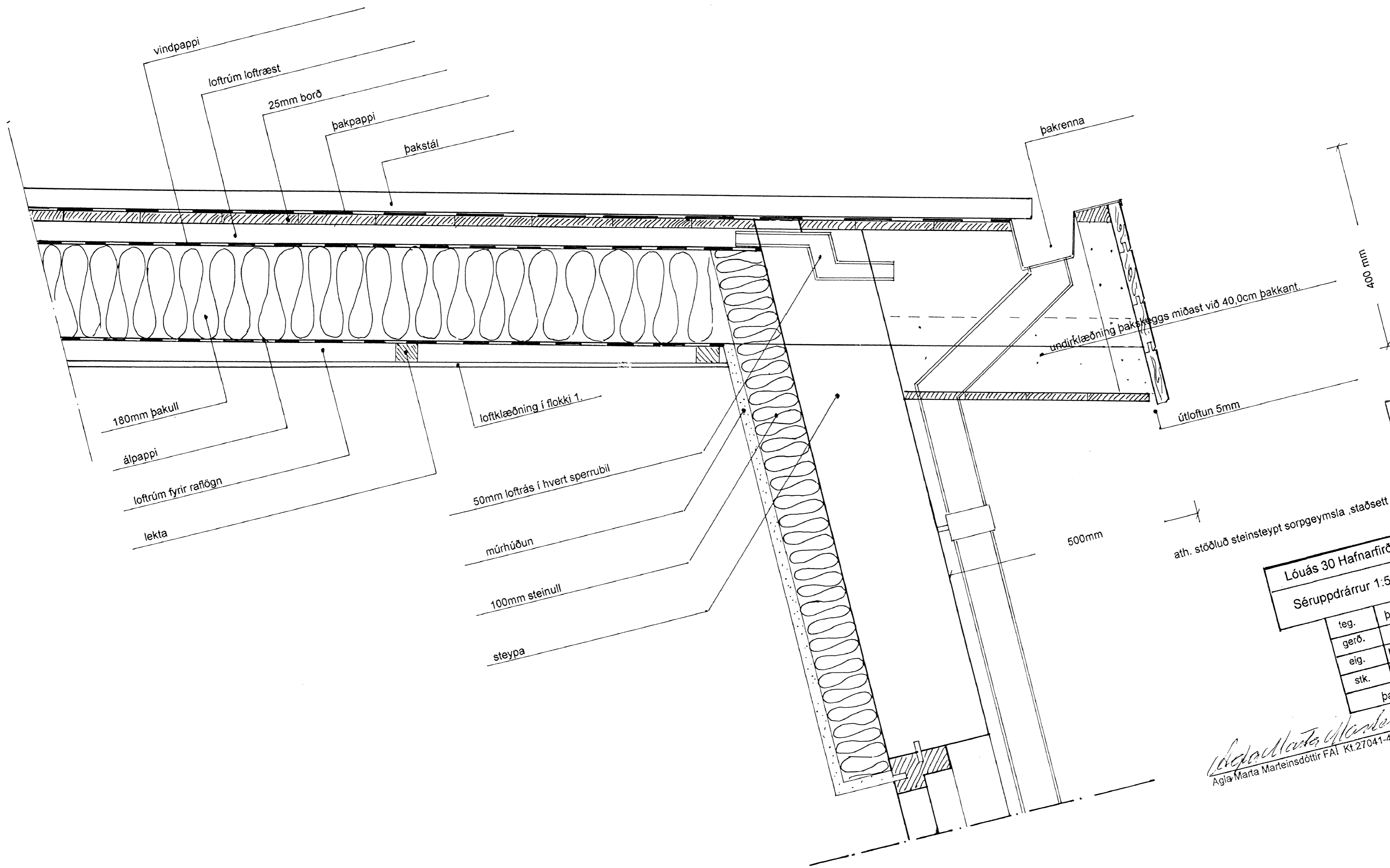
sneiðing af þakbrún 1:5
